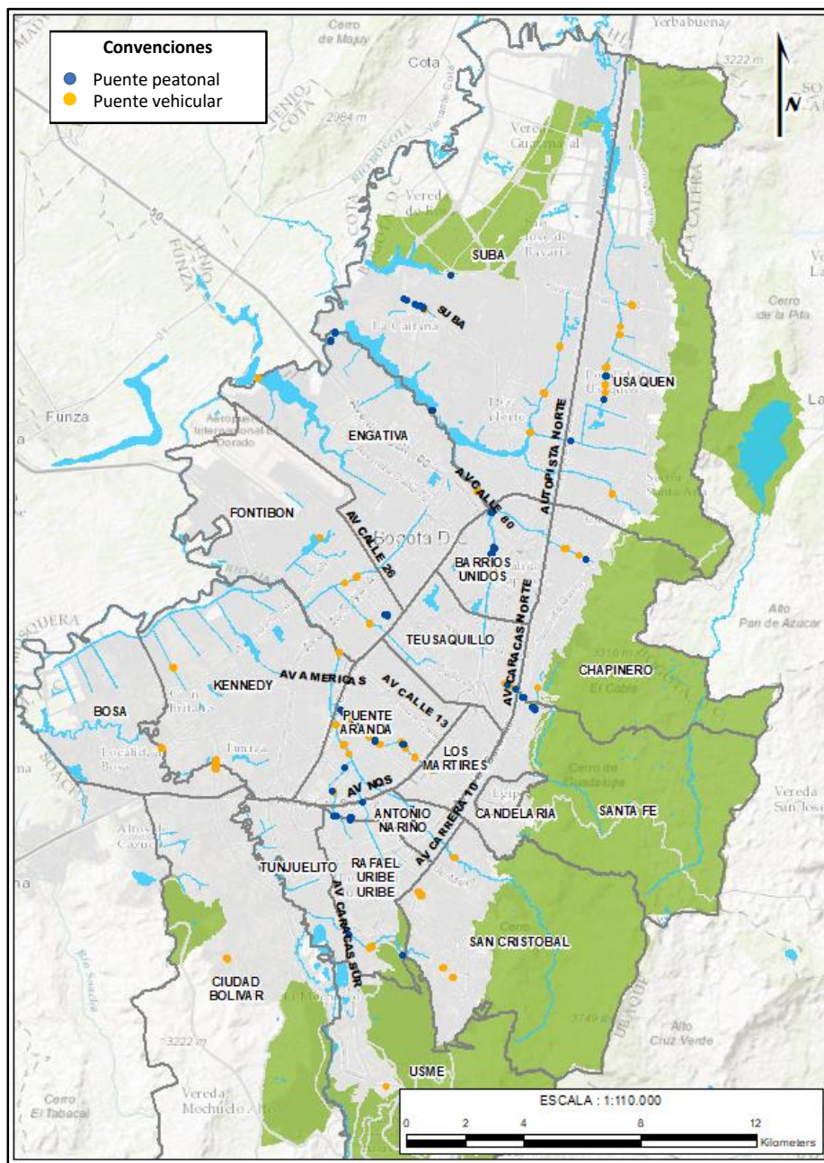
Mapa 13. Inventario de puentes del Distrito por malla vial intermedia
