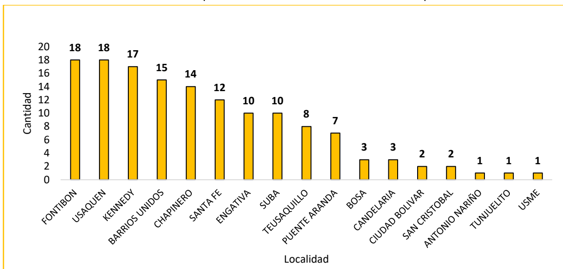
Gráfica 9. Inventario de puentes vehiculares del Distrito sobre vía por Localidad
