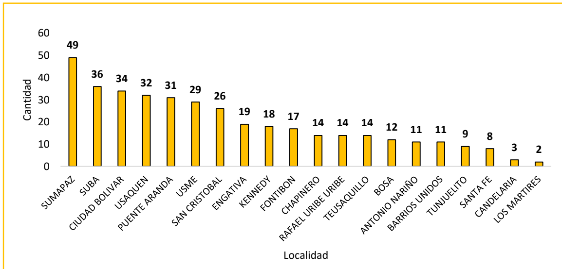
Gráfica 10. Inventario de puentes vehiculares del Distrito sobre cuerpo de agua por Localidad
