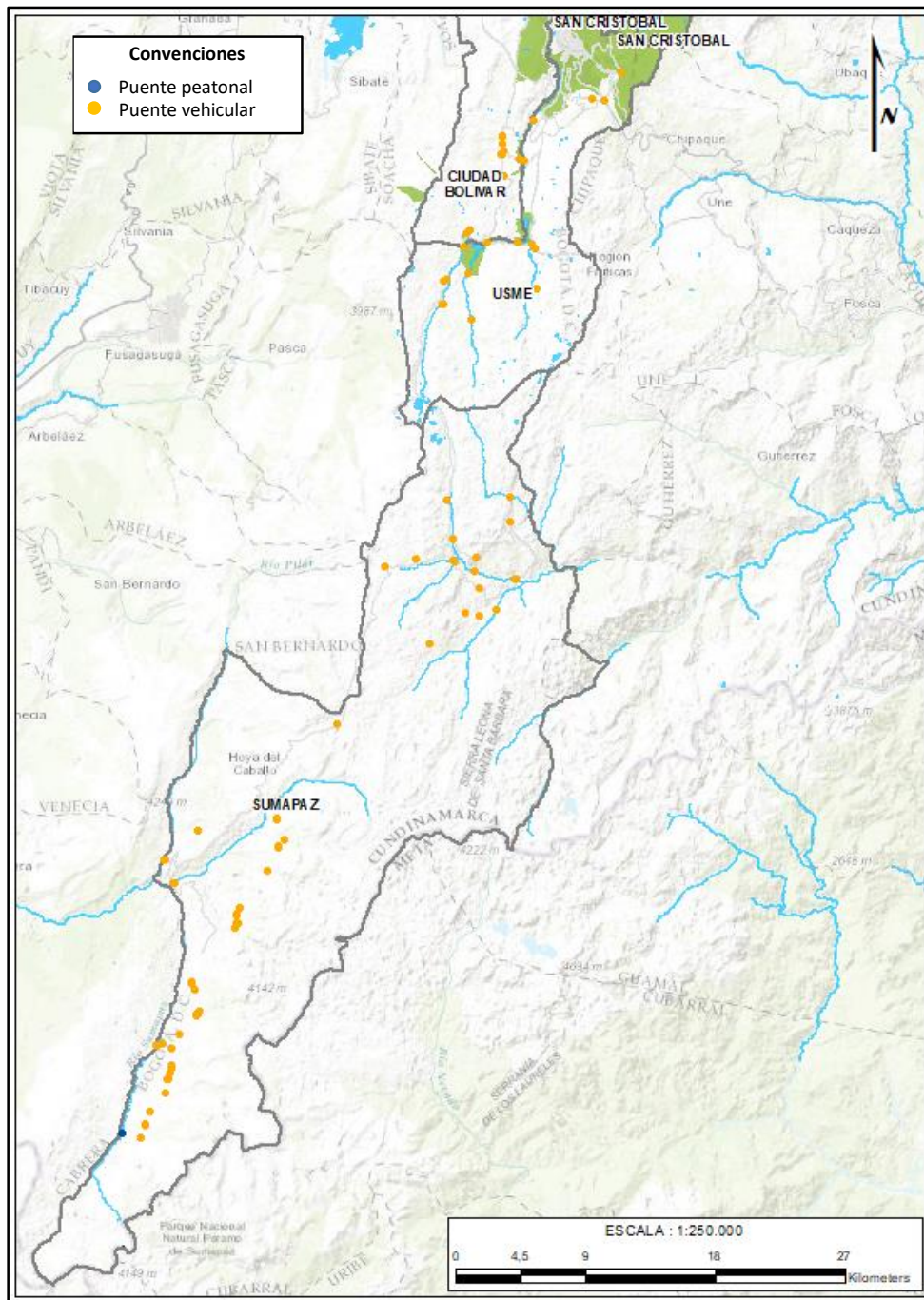
Mapa 17. Inventario Puentes del Distrito por uso del suelo rural
