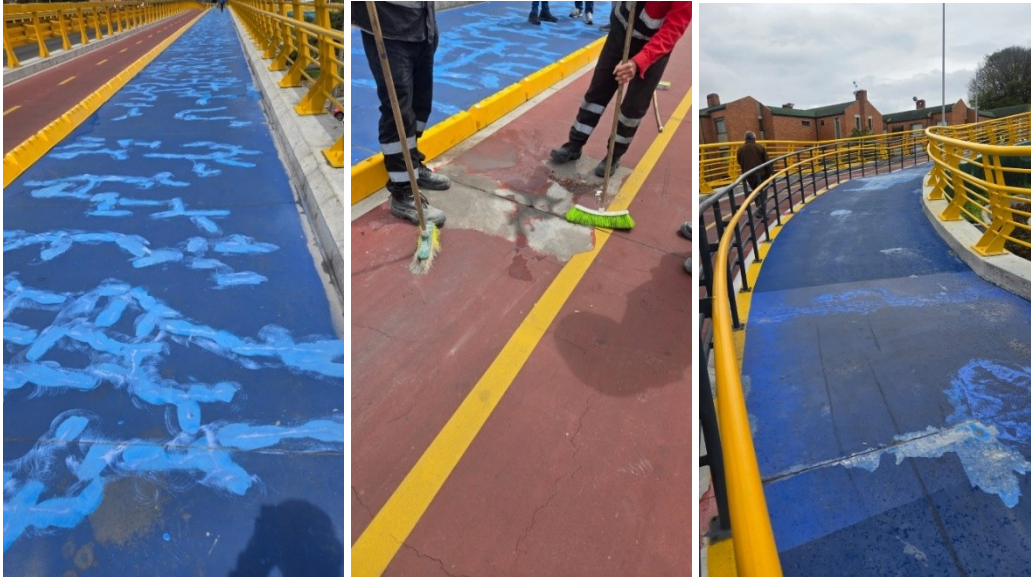
Imagen 7 – 8 – 9. – Intervención paso peatonal tablero puente. Fuente Propia
