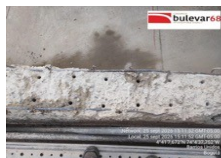
Ilustración Perforación en pantallas existentes C, D y E
