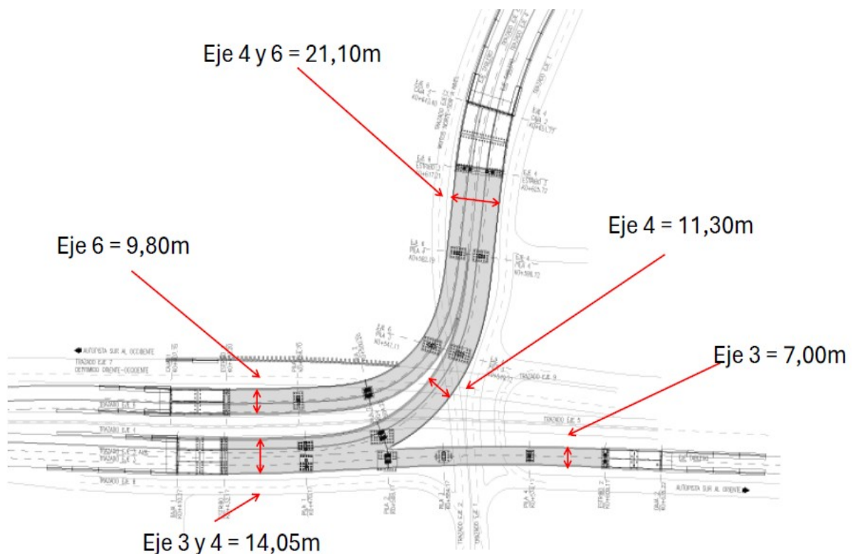
Diseño geométrico nuevos puentes de Venecia
