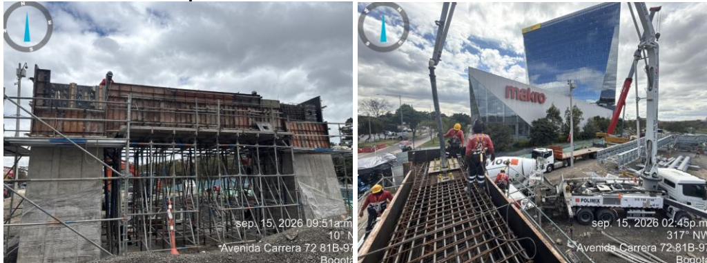
Fotografía N°1: Enconfrado y vaciado de viga riostra entre Columnas de apoyo principal de pasarela central en el costado occidental.
