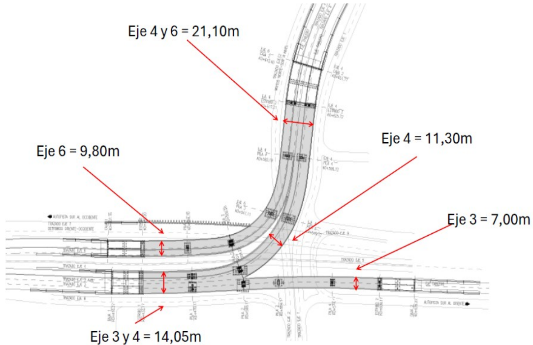
Diseño geométrico nuevos puentes de Venecia
