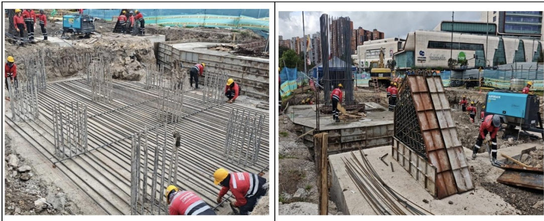
Fotografía N°1: Actividades de obra de cimentación y montaje.
