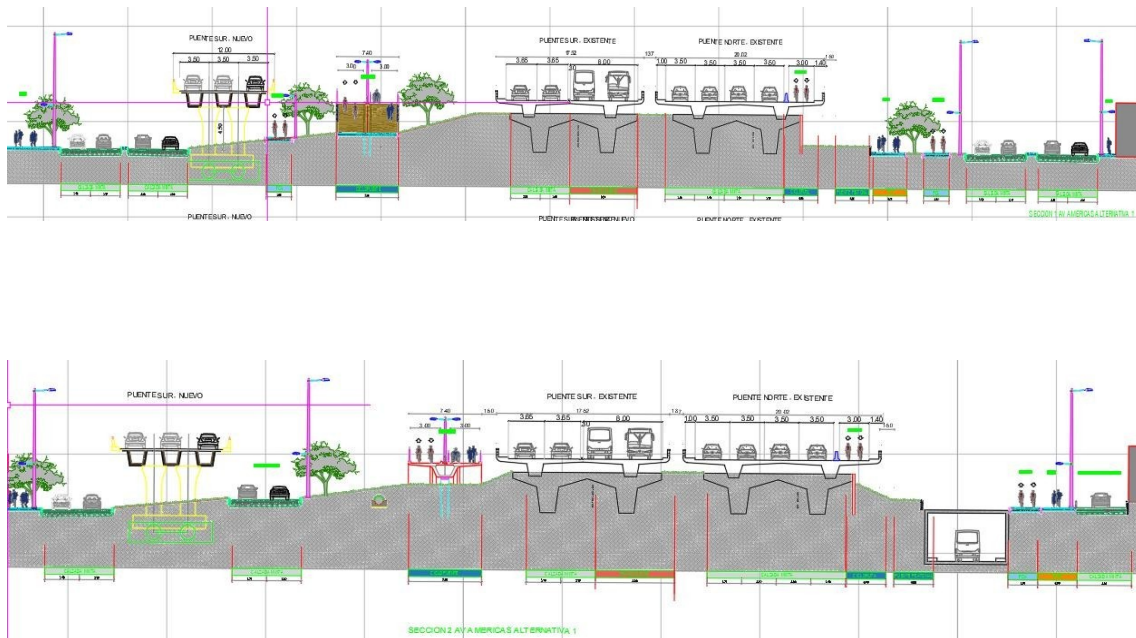
SECCIONES TRANSVERSALES AV. AMÉRICAS CON AV. CARRERA 68. (A la izquierda el costado sur). Fuente: Contrato IDU No. 529 de 2022.
