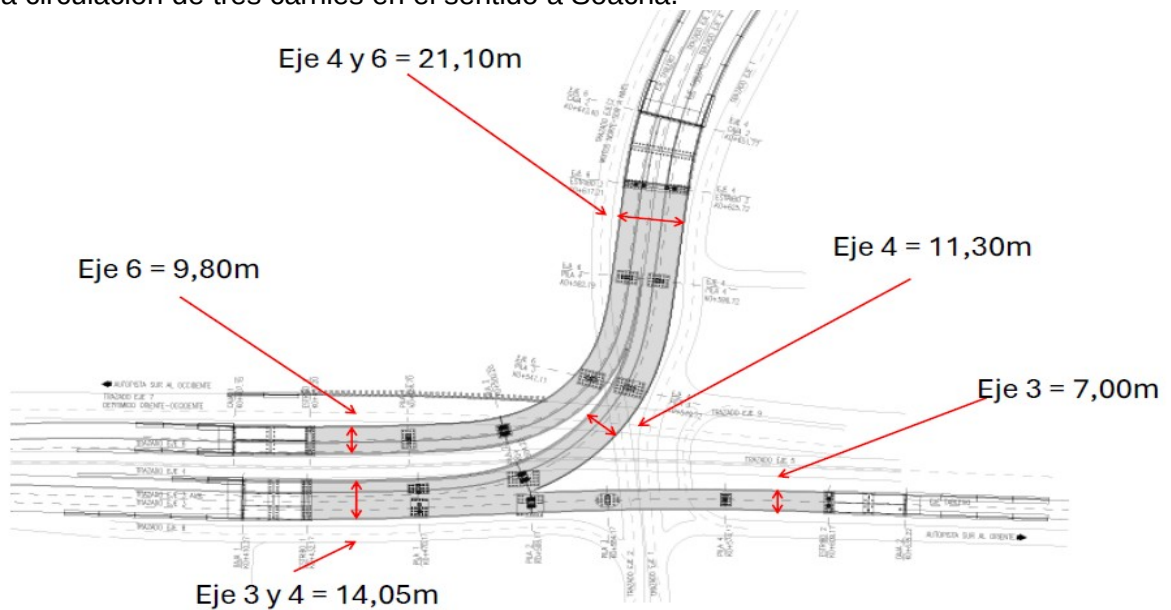
Diseño geométrico puentes de Venecia
