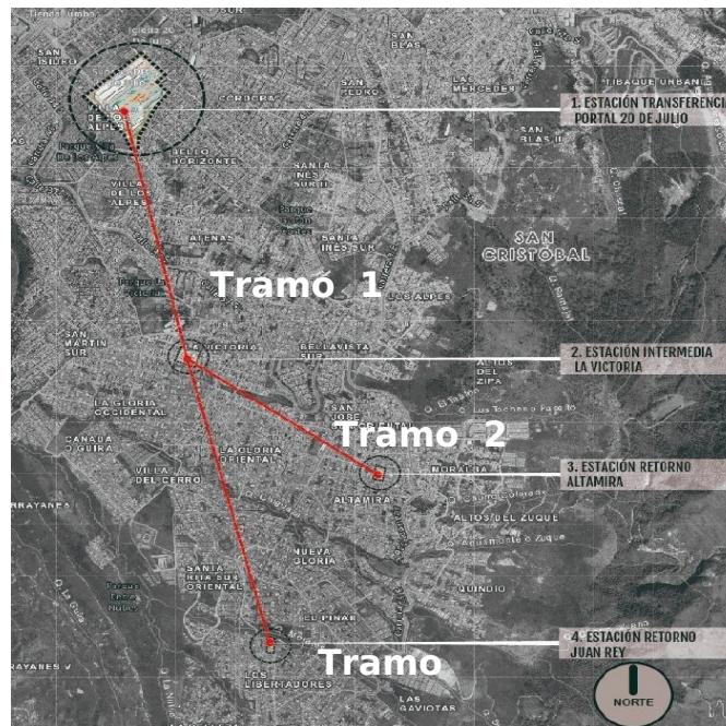
Figura 1. Localización de los tres tramos del corredor de Cable Aéreo San Cristóbal
