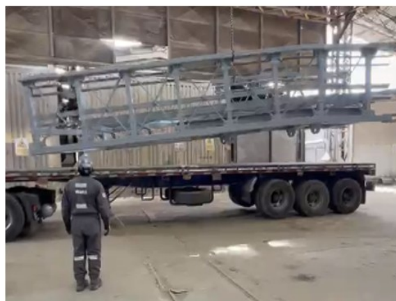
Fotografía N°3: Cargue y traslado de Estructura metálica desde la planta de producción hacia los frentes de obra.
