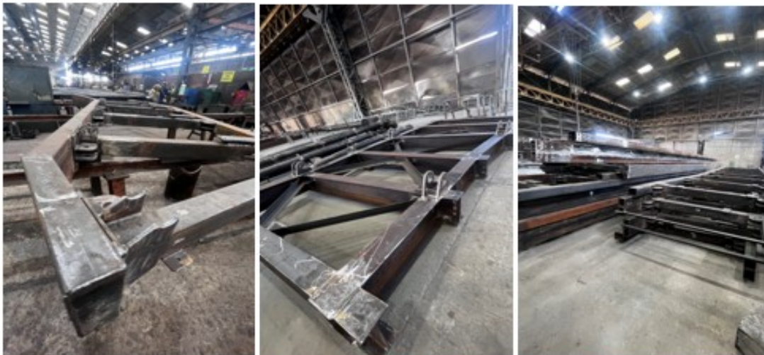
Fotografía N°3: Avance de Estructura Metálica, en visita a planta el 17/06/2026.
