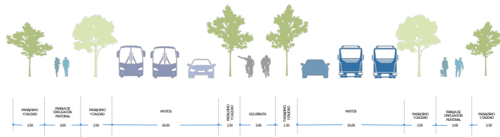
Ilustración 2 Perfil vial propuesto.
