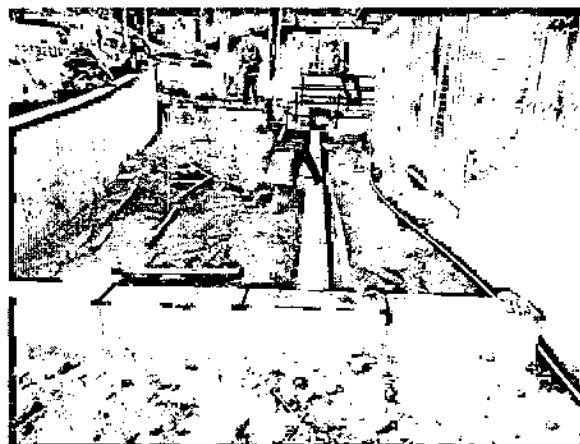
Ilustración 30. Instalación Bordillos A-80 conformación Andenes en el Barrio Altos del Virrey
