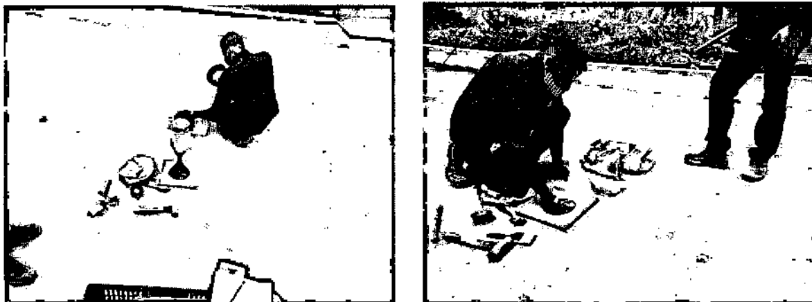
Ilustración 56. TOMA DE DENSIDADES CONO DE ARENA
