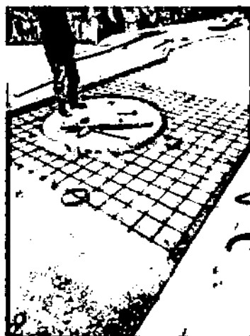
Ilustración 16. Acero de Refuerzo Tapa Colector y Empalmes Vía en el Barrio Altamira
