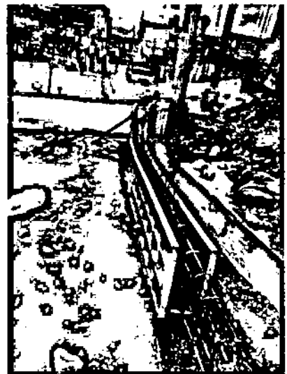
Ilustración 11. Acero de Refuerzo Muros en el Barrio Altamira
