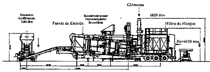
Figura 1. Dimensiones de la planta de mezclas asfálticas. Fuente: SOFAN INGENIERÍA S.A.S.
