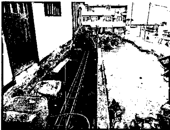
Ilustración 24. Acero de Refuerzo Muro en Anden CIV 4007971
