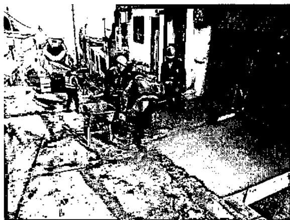
Ilustración 40. Fundida de Rampa y Muros CIV 4007972
