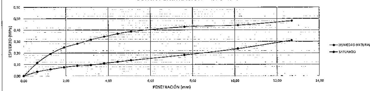
CURVA PENETRACIÓN - ESFUERZO
