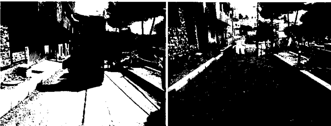
Ilustración 11. COMPACTACION DE SUBBASE GRANULAR CLASE C (TRAMO 2 – EMPALME VIA) CIV 4005352
