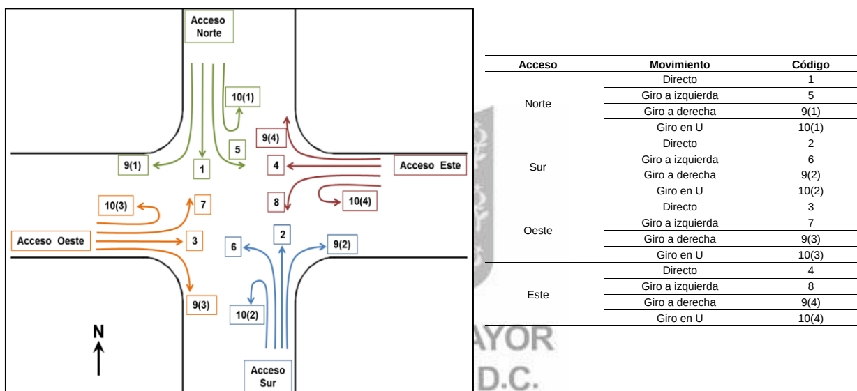
Figura 6-7. Representación esquemática de los movimientos en una intersección
