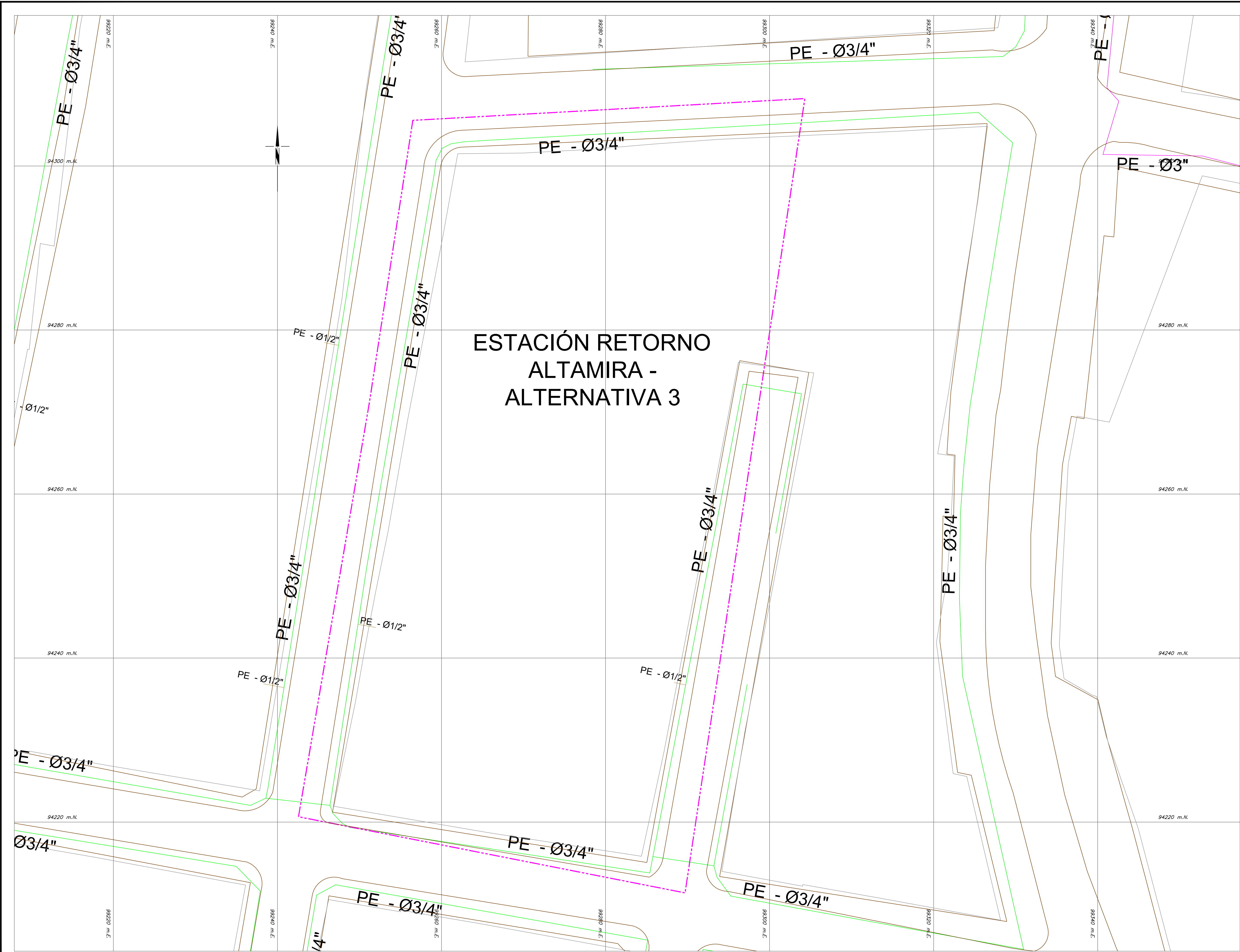
PLANTA GENERAL ESCALA: 1:200
