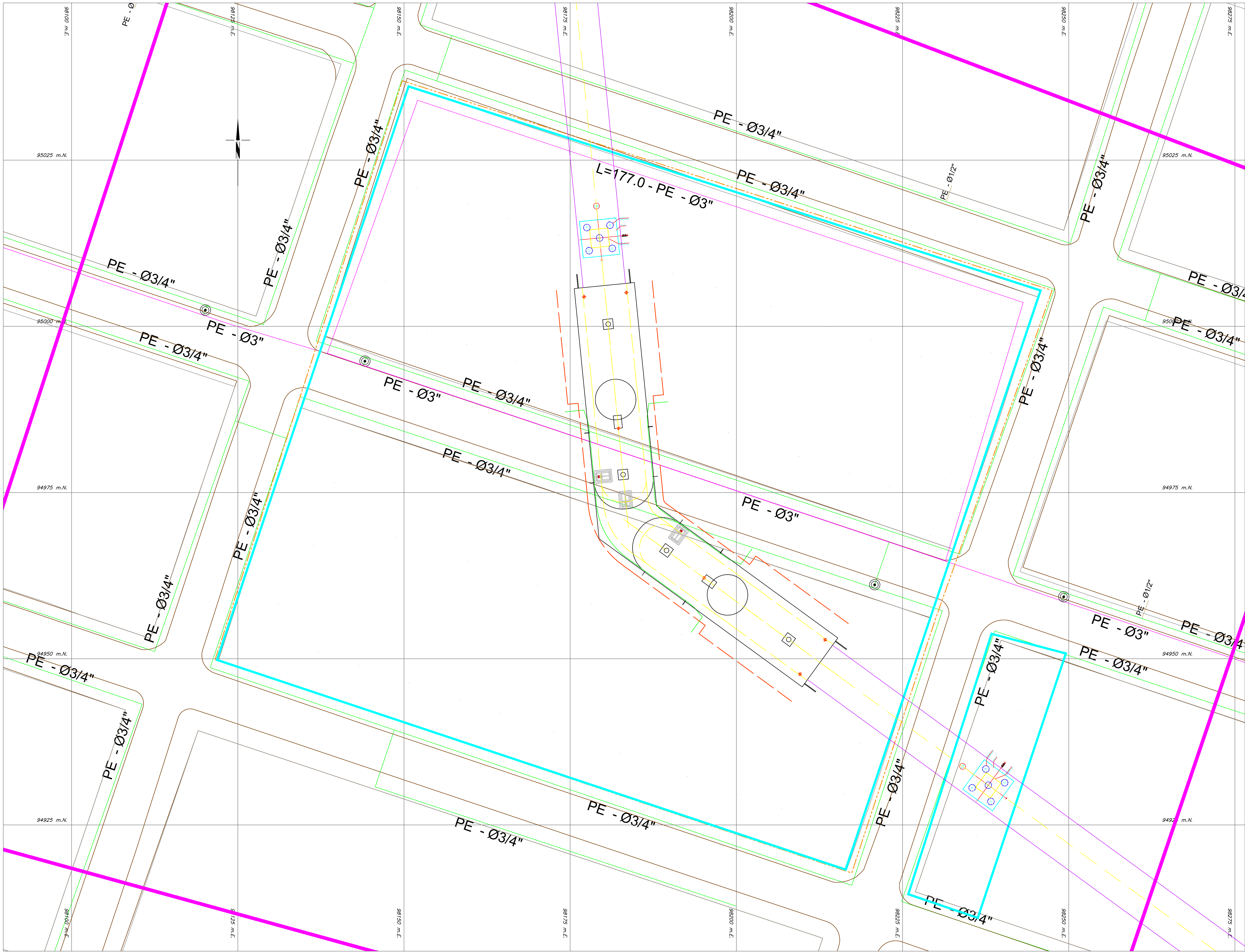
PLANTA GENERAL ESCALA: 1:250
