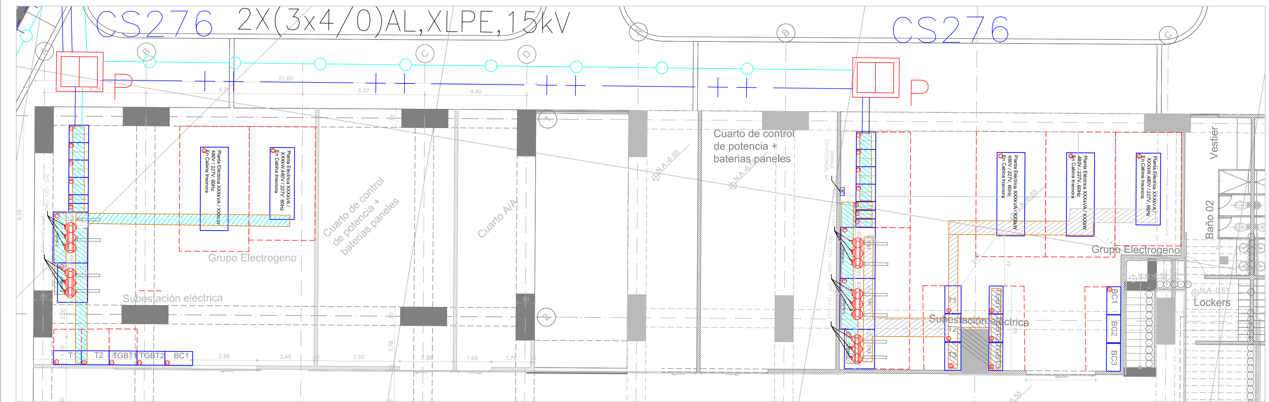
DETALLE EN PLANTA SUBESTACION ESCALA - 1:100
