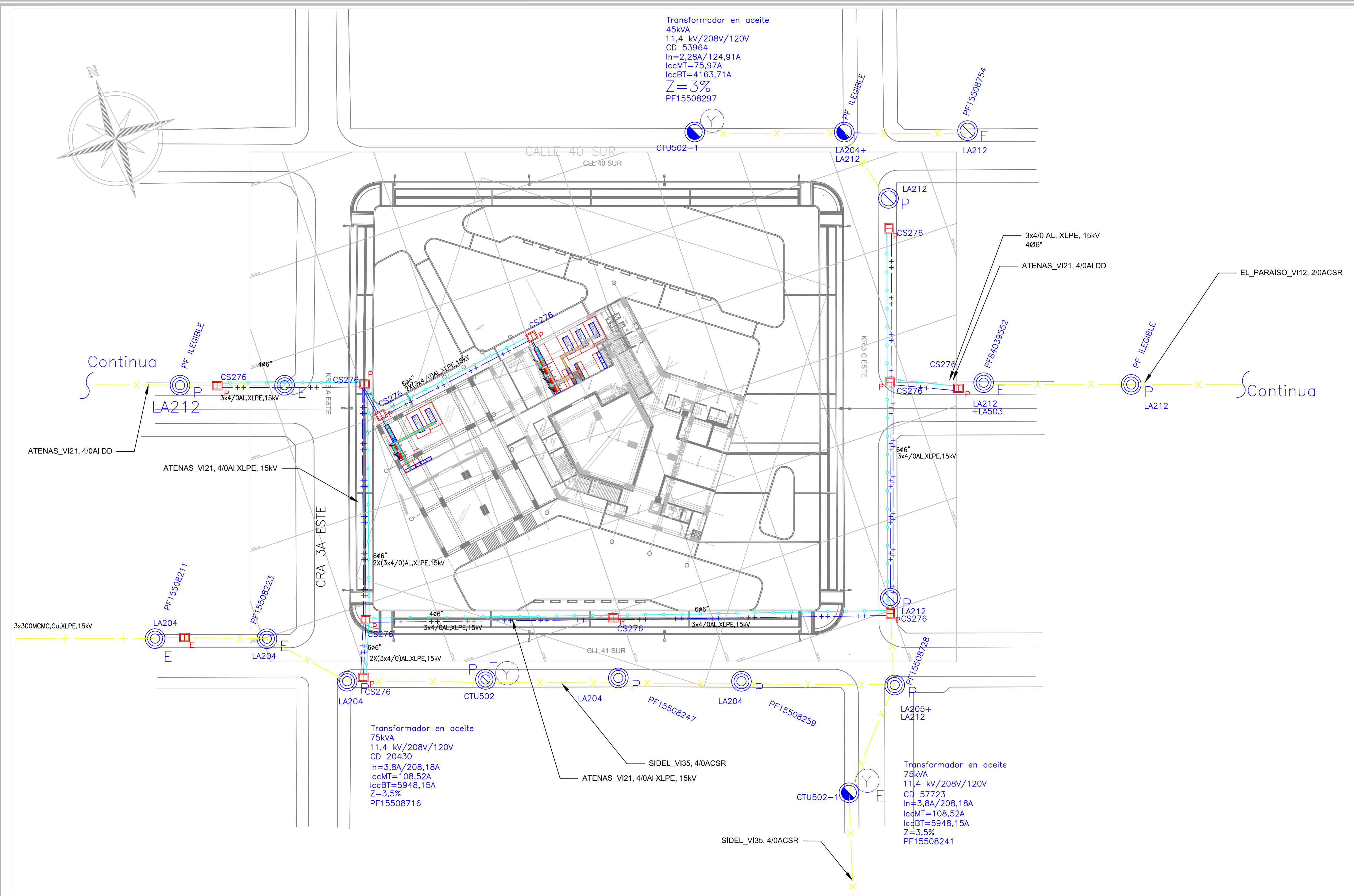
PLANTA RED M.T. PROYECTADA ESCALA - 1:500
