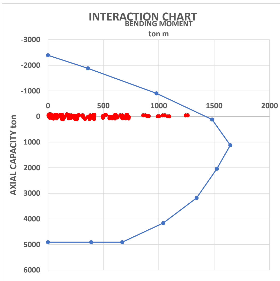
Figura 10.3 – Diagrama de interacción mástil
