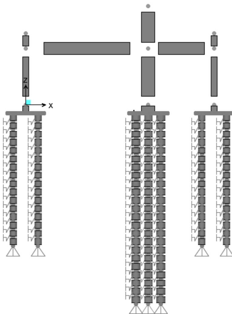
Figura 8.2 – Elevación modelo de análisis SAP2000
