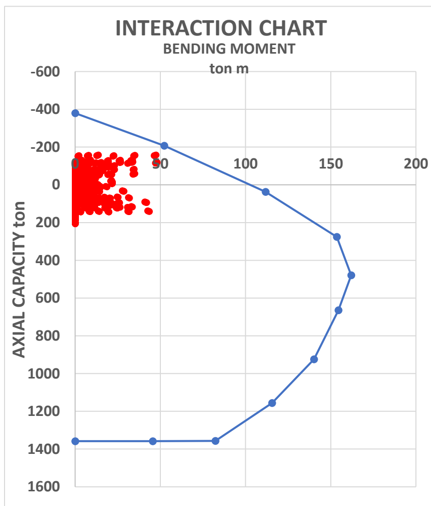
Figura 10.2 – Diagrama de interacción pilas
