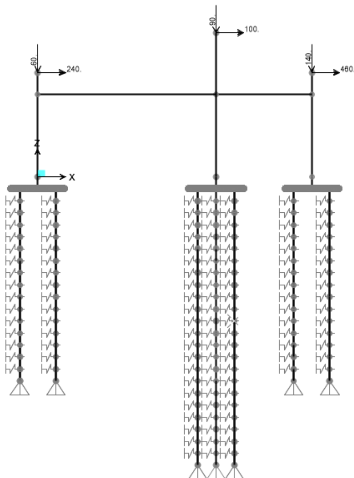
Figura 12.2 – Cargas Variables (vehículo en operación), en KN
