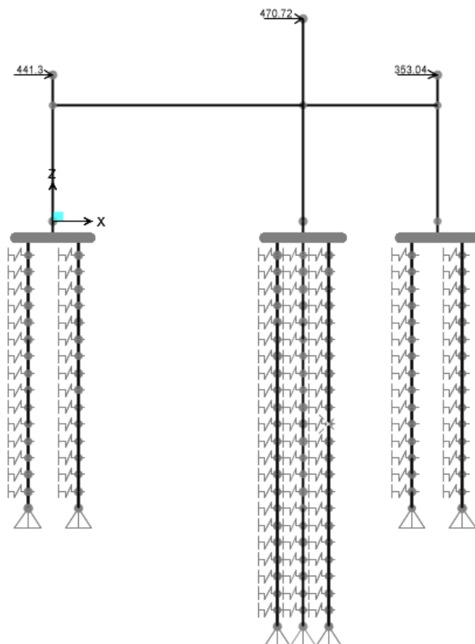
Figura 12.3 – Cargas Accidentales (sismo X), KN
