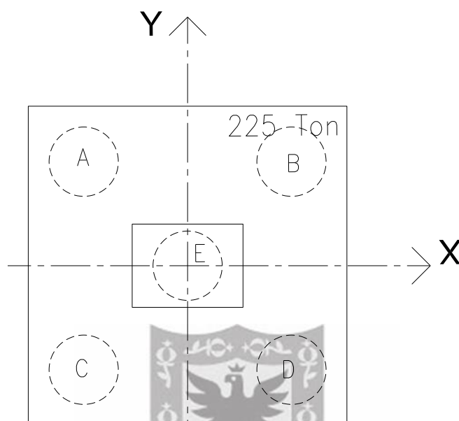
Figura 10.1 – Planta cimentación descarga máxima
