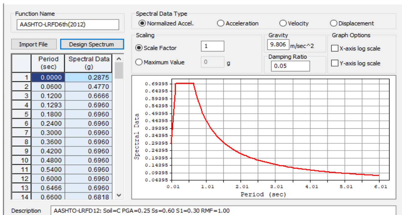
DE BOGOTÁ D.C. Figura 6.1 – Espectro sísmico de diseño Instituto de Desarrollo Urbano
