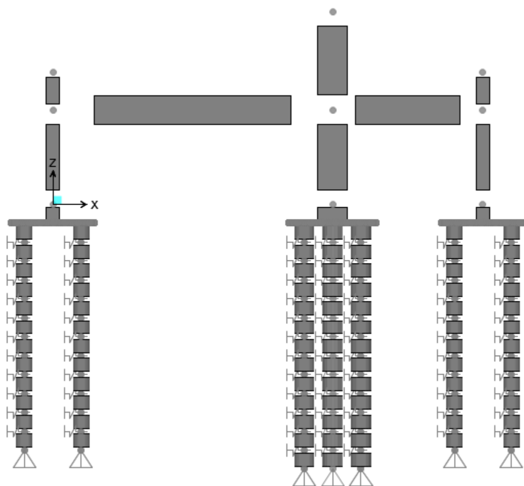
Figura 8.2 – Elevación modelo de análisis SAP2000
