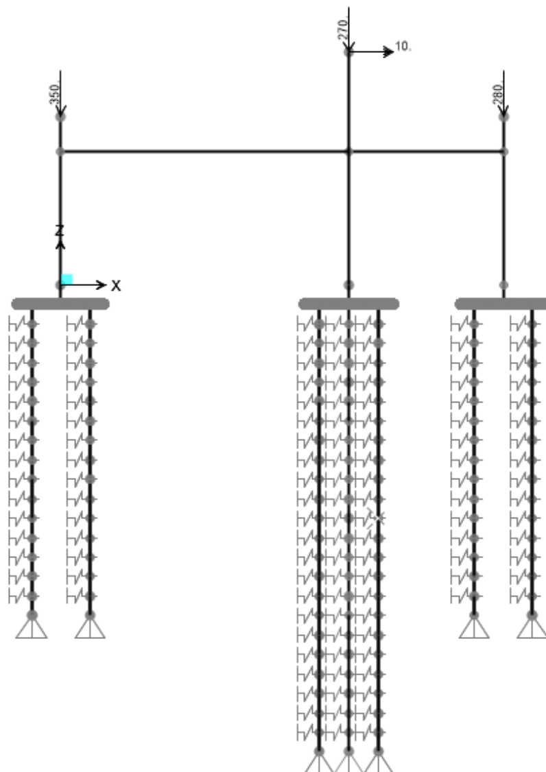
Figura 12.1 – Cargas Permanentes (peso estación), KN
