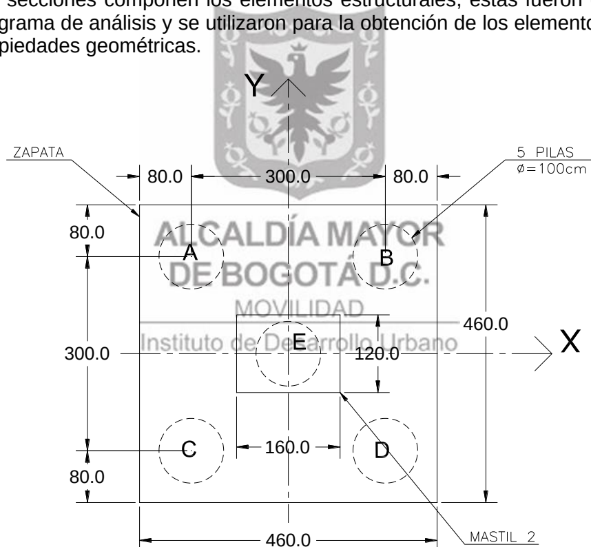
Figura 8.1 – Planta cimentación mástil 2
