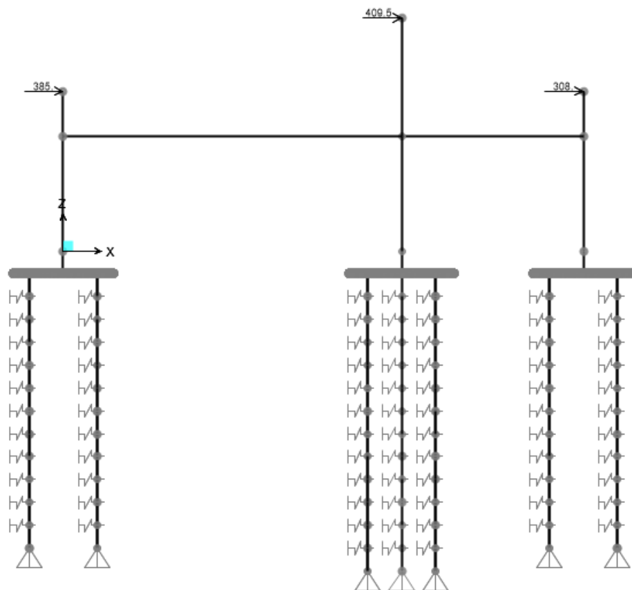
Figura 12.3 – Cargas Accidentales (Sismo dirección X), KN
