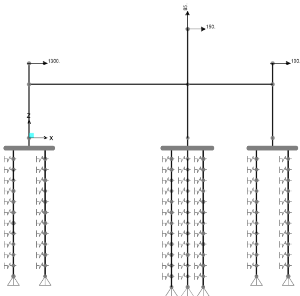
Figura 12.2 – Cargas Variables (Viento Lateral fuera de operación), KN
