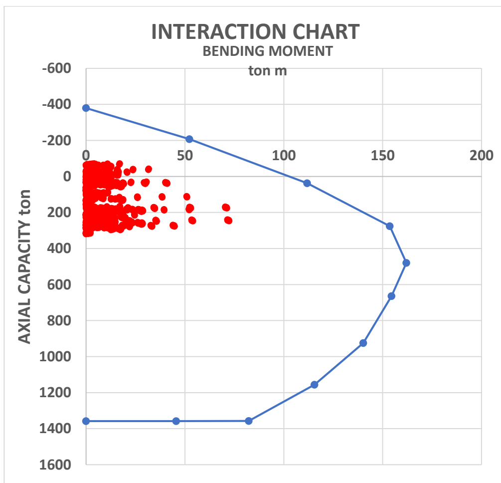
Figura 10.2 – Diagrama de interacción pilas
