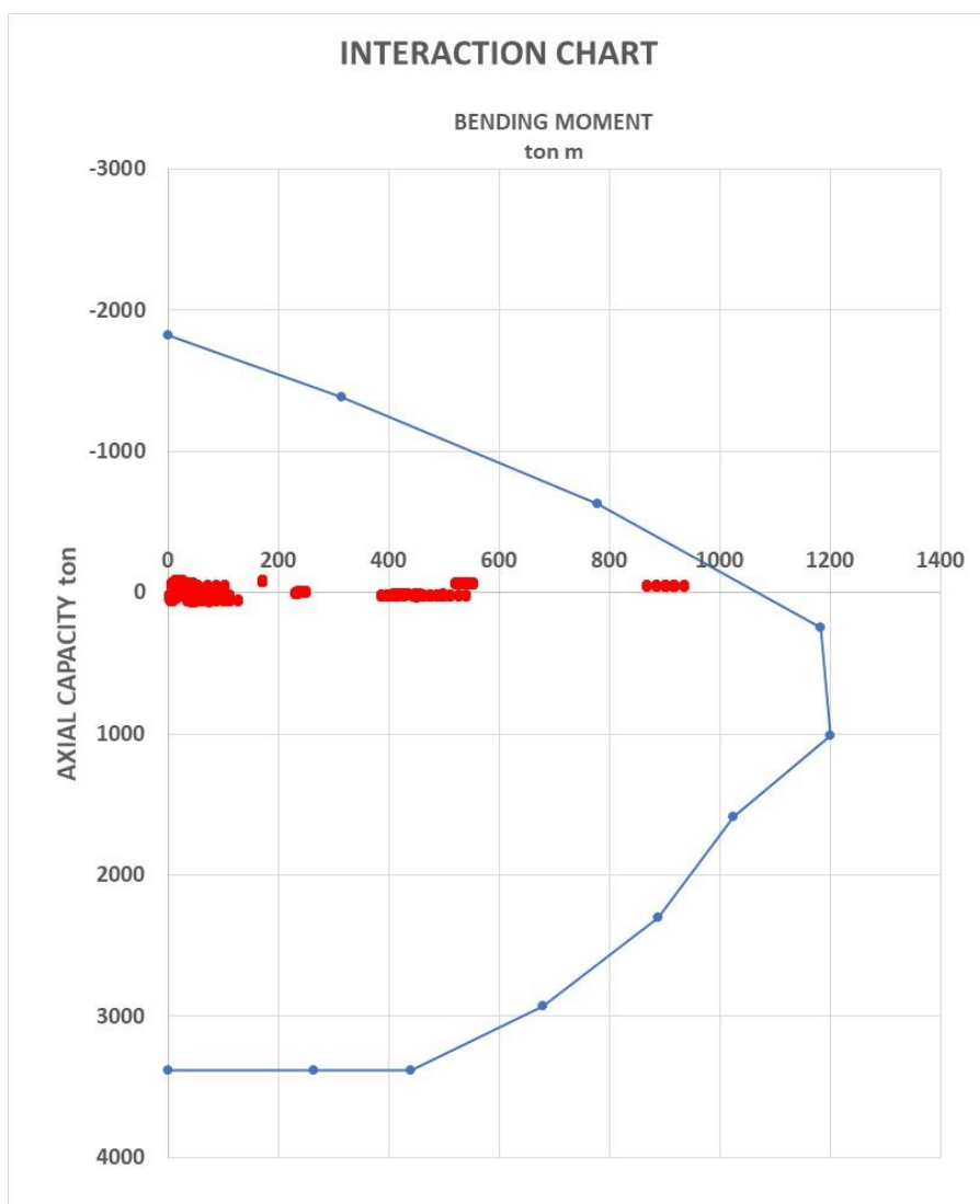
Figura 10.3 – Diagrama de interacción mástil
