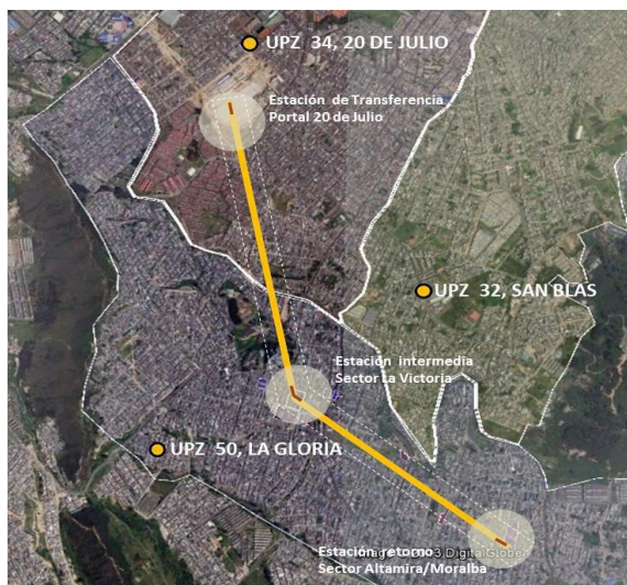
Figura 2.1 – Trazo cable aéreo
