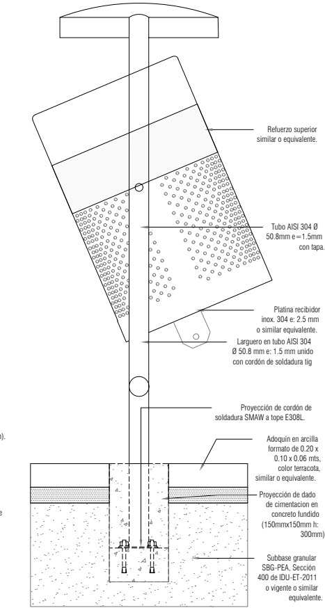
ESC: 1:10 06-ALZADO: PAPELERA DOBLE EN ACERO
