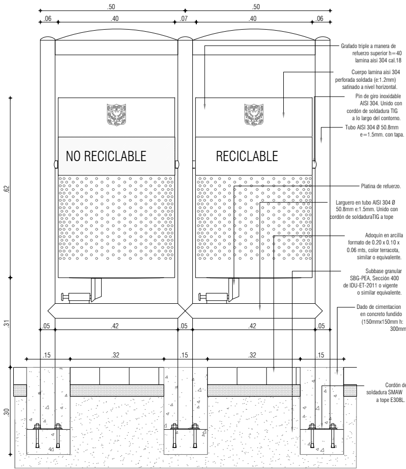
03-ALZADO: PAPELERA DOBLE EN ACERO EN ZONA DURA ESC.1:10
