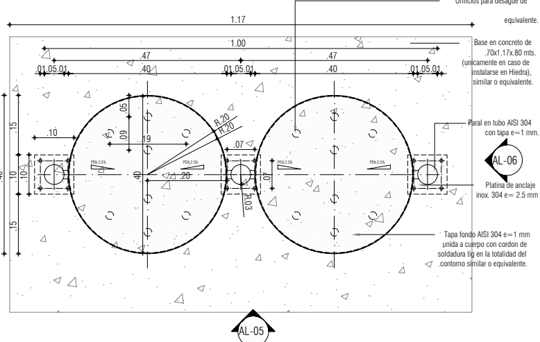
PLANTA: PAPELERA DOBLE EN ACERO EN ZONA VERDE ESC: 1:10
