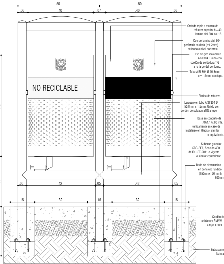
04-ALZADO: PAPELERA DOBLE EN ACERO 05-ALZADO: PAPELERA DOBLE EN ACERO ZONA VERDE ESC: 1:10
