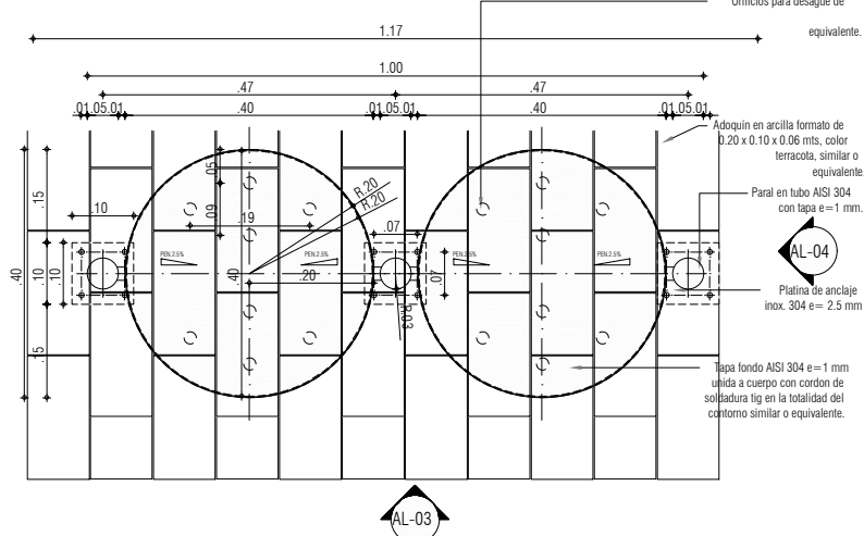
PLANTA: PAPELERA DOBLE EN ACERO EN ZONA DURA ESC:1:10
