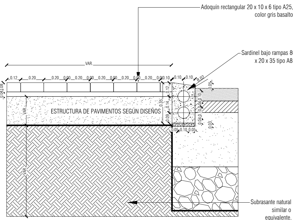
CORTE A-A DETALLE SARDINEL BAJO RAMPAS A-85 ESC: 1:20
