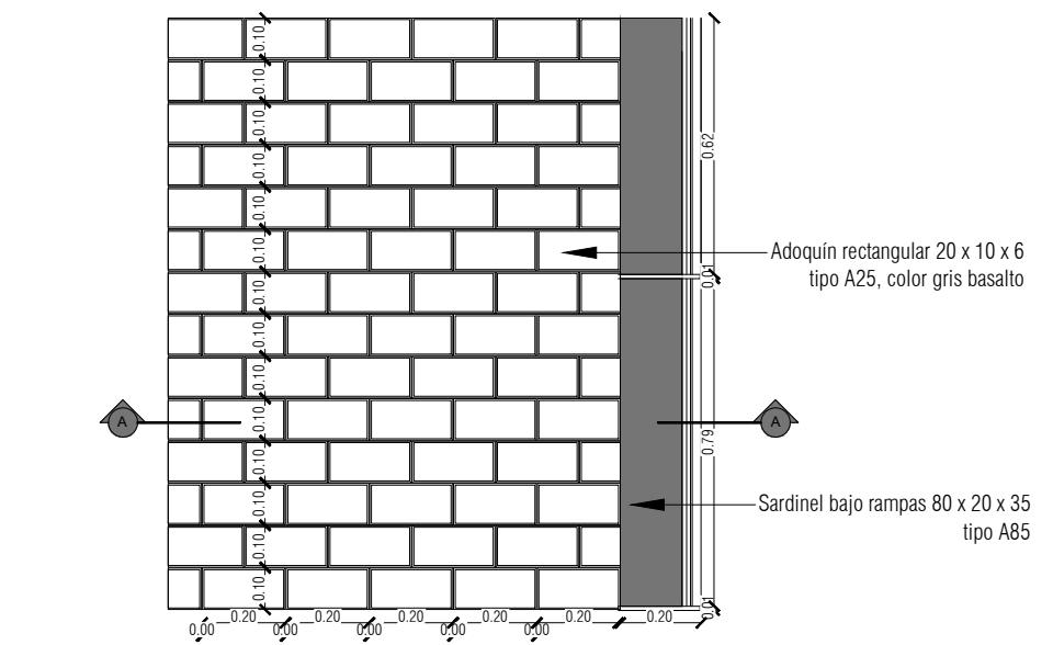
PLANTA DETALLE SARDINEL BAJO RAMPAS A-85 ESC: 1:20
