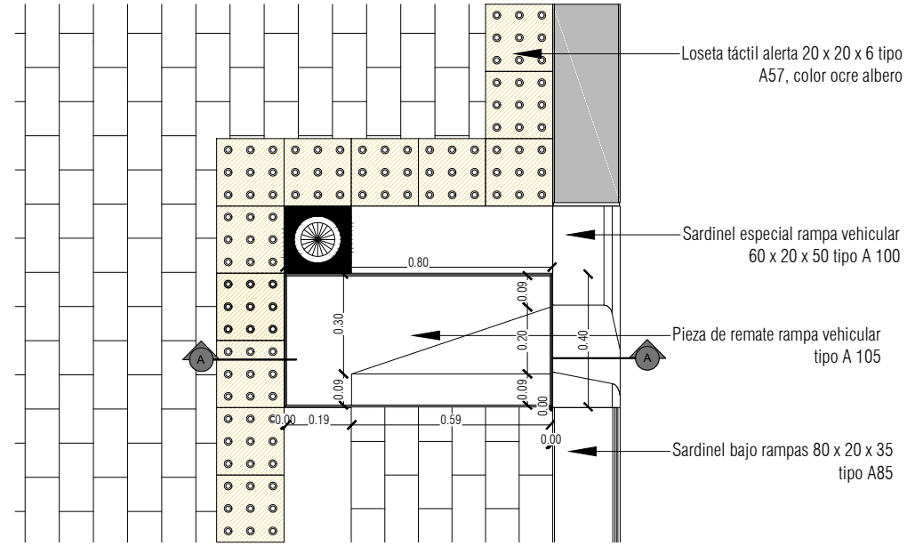
PLANTA PIEZA REMATE ESPECIAL RAMPA A-105 ESC: 1:20
