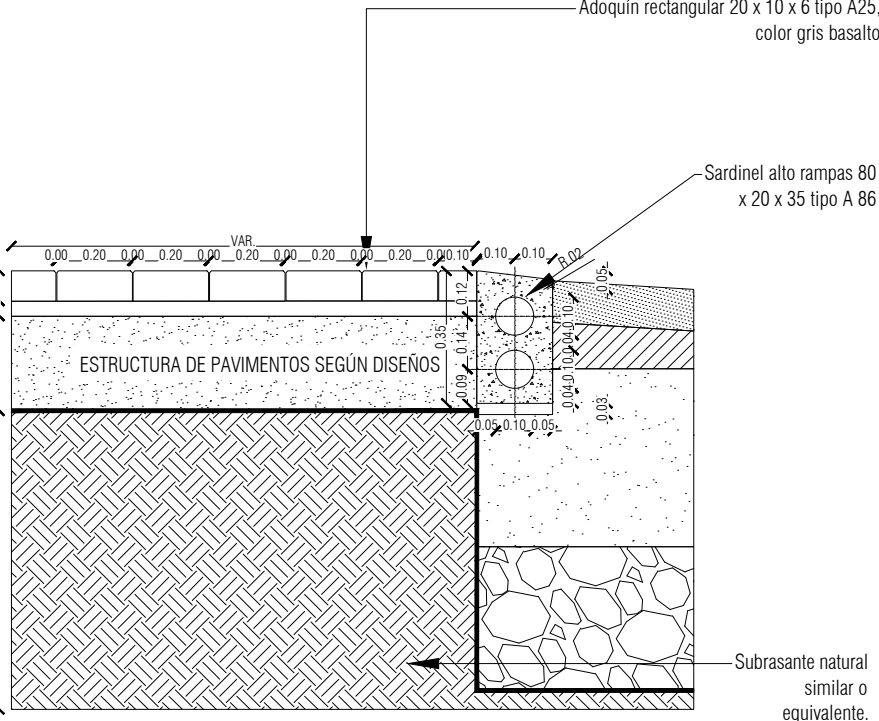
CORTE A-A DETALLE SARDINEL ALTO RAMPAS A-86 ESC: 1:20
