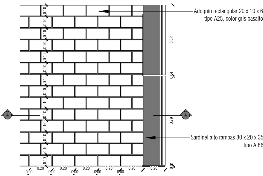
PLANTA DETALLE SARDINEL ALTO RAMPAS A-86 ESC: 1:20
