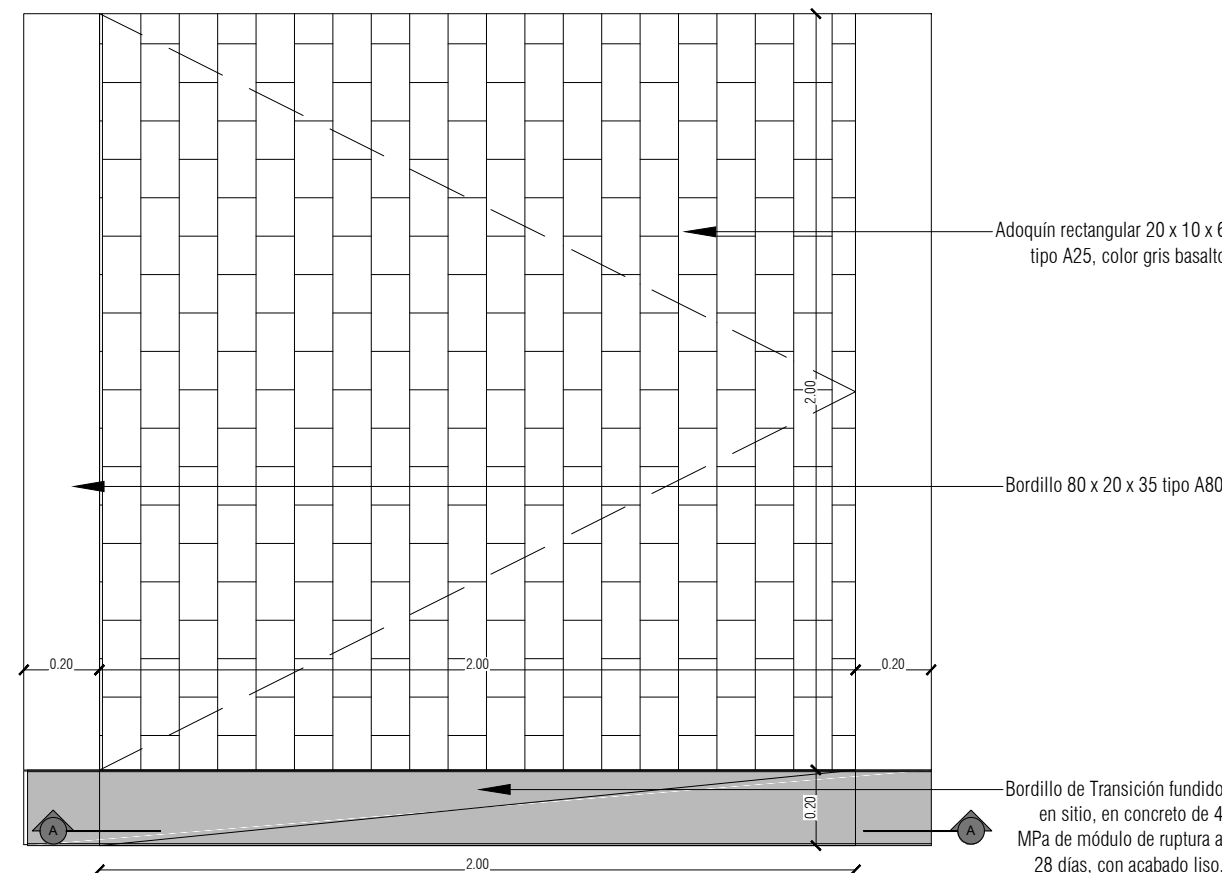
PLANTA DETALLE BORDILLO DE TRANSICION PIEZA REMATE RAMPA ENTRE SARDINEL ALTO A-86 Y SARDINEL BAJO A-85 ESC: 1:20
