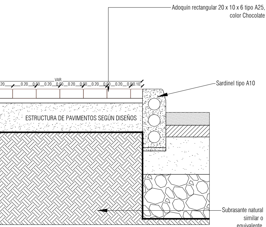
RTE A-A DETALLE ADOQUÍN A-25 -CHOCOLATE ESC: 1:20
