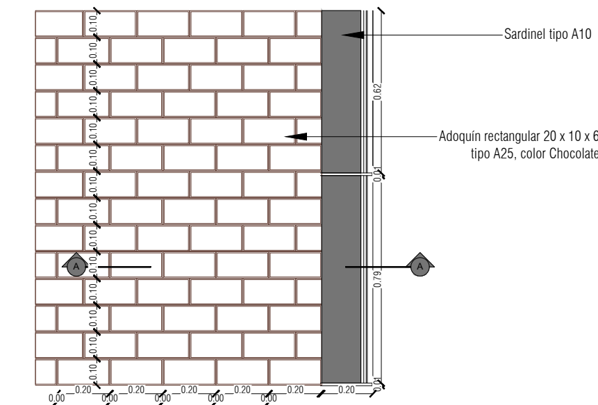
PLANTA DETALLE ADOQUÍN A-25 -CHOCOLATE ESC: 1:20
