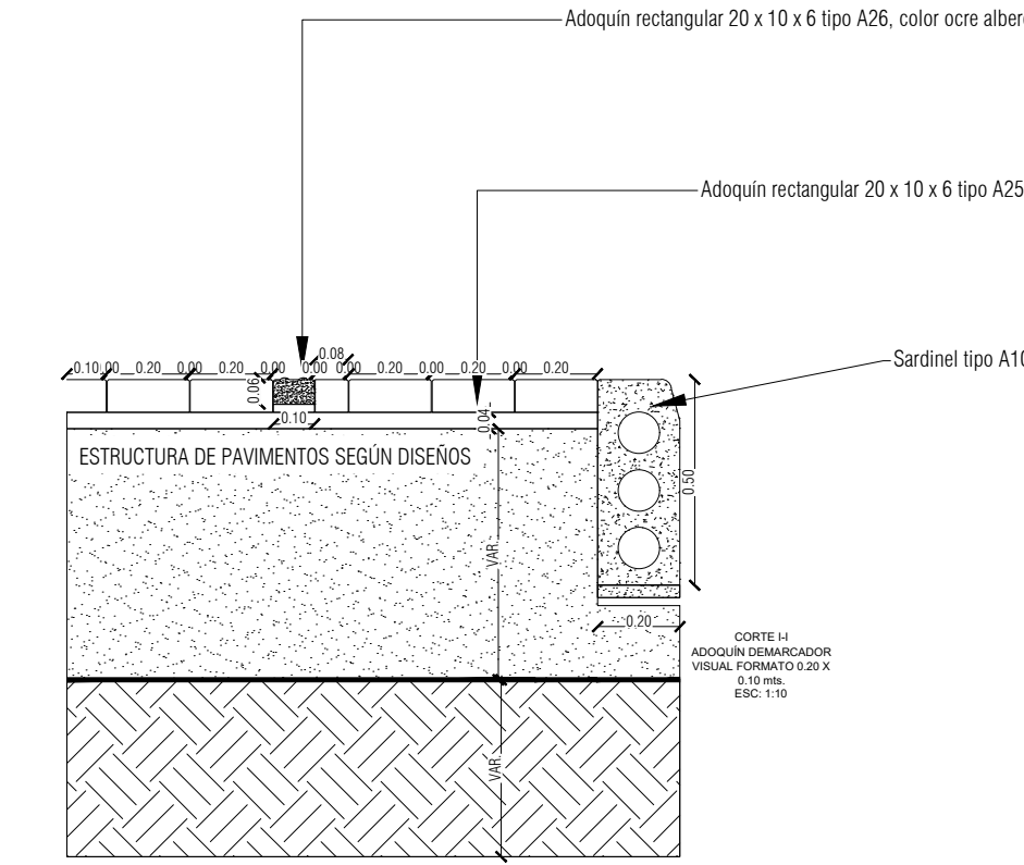
PLANTA DETALLE ADOQUÍN A-26 TACTIL ALERTA -OCRE ALBERO ESC: 1:20
