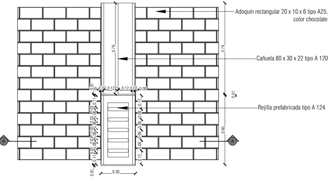
PLANTA REJILLA CAÑUELA PREFABRICADA TIPO A-124 ESC 1 : 20
