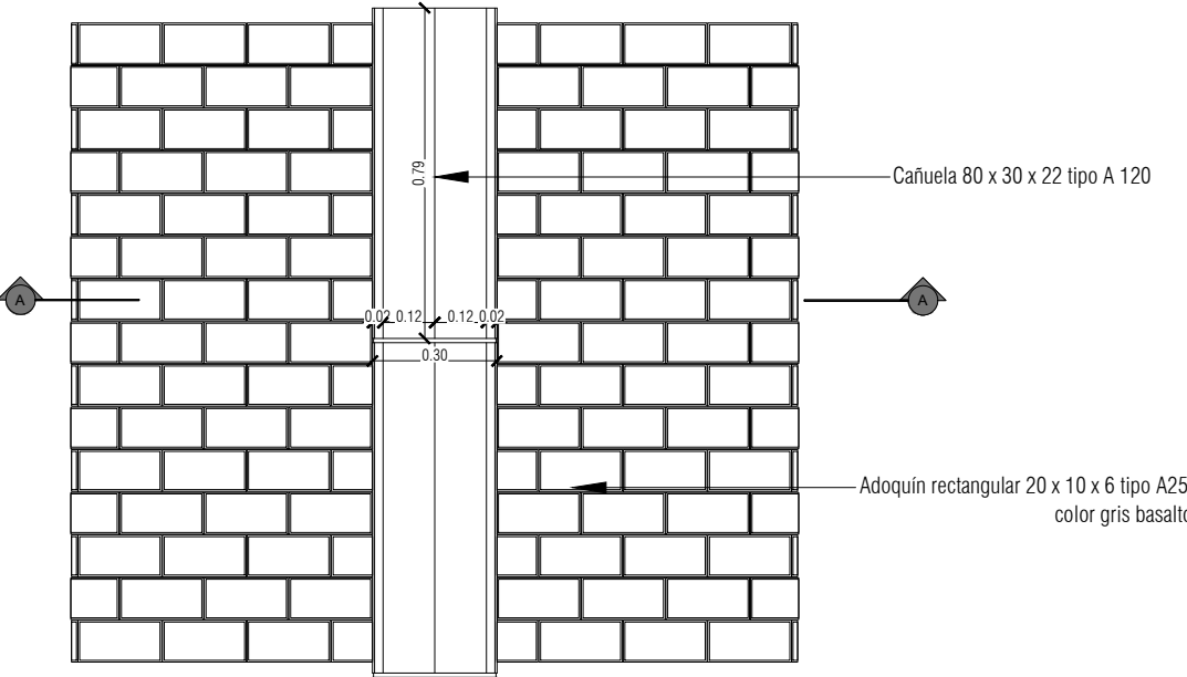
PLANTA CAÑUELA PREFABRICADA TIPO A120 ESC 1 : 20
