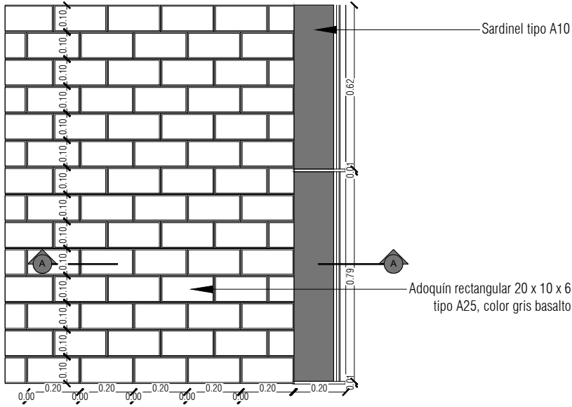
PLANTA DETALLE ADOQUÍN A-25 -GRIS ESC: 1:20
