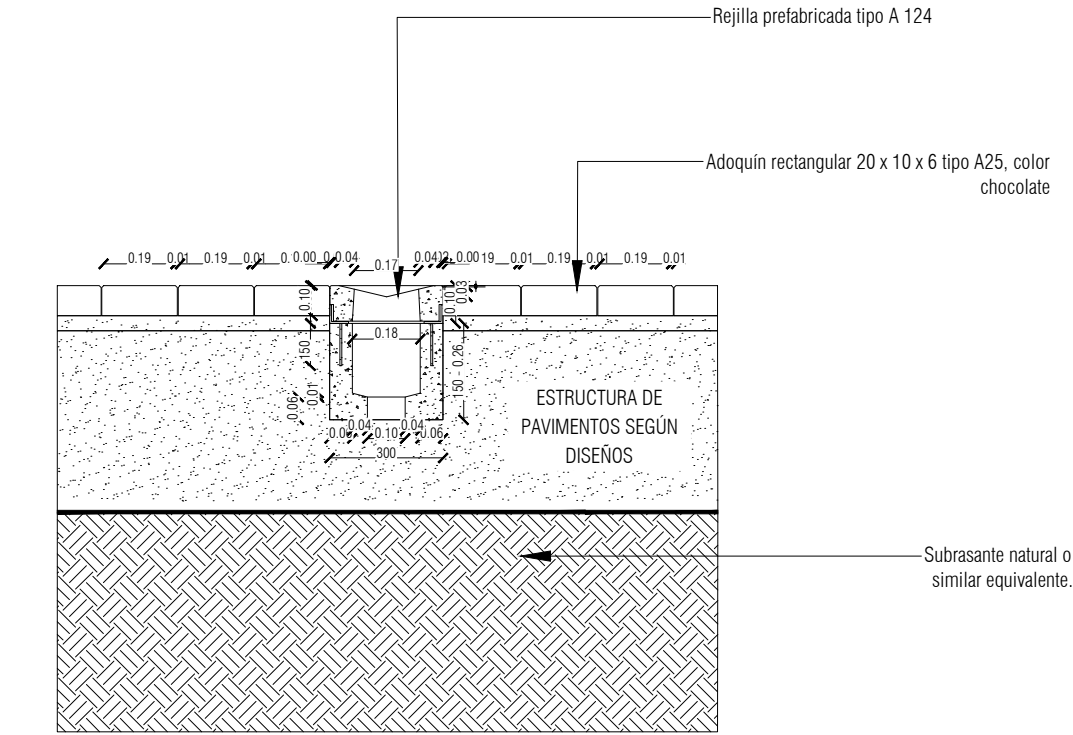
CORTE A-A CAÑUELA PREFABRICADA TIPO A-124 ESC 1 : 20
