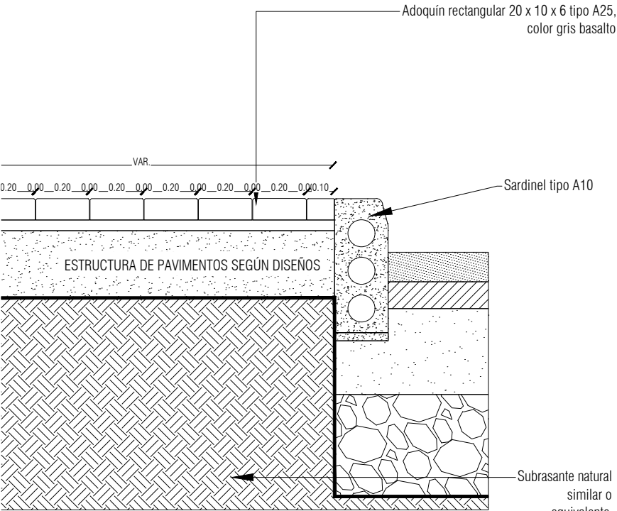
ORTE A-A DETALLE ADOQUÍN A-25 -GRIS ESC: 1:20
