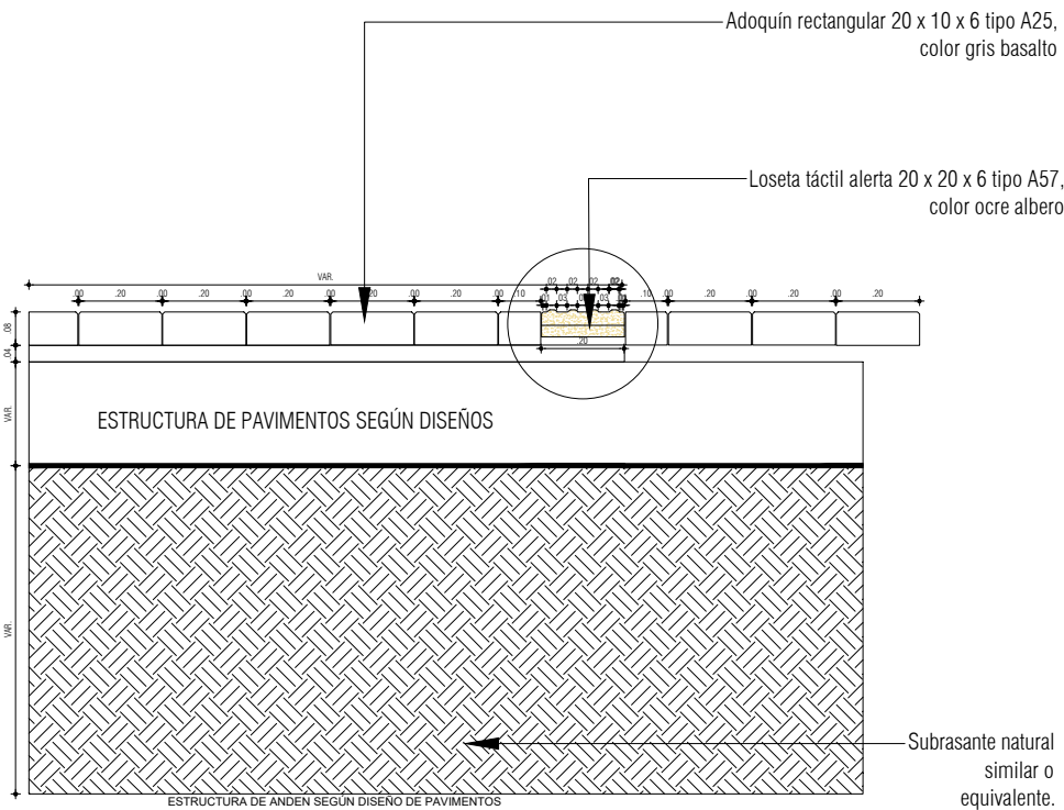
CORTE A-A DETALLE LOSETA A-57 ESC: 1:20
