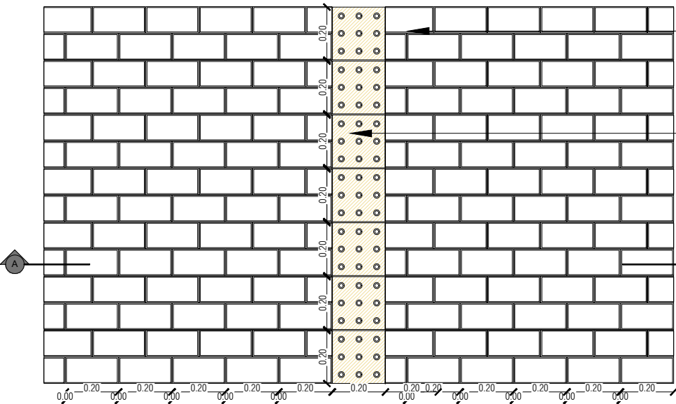
PLANTA DETALLE LOSETA A -57 ESC: 1:20
