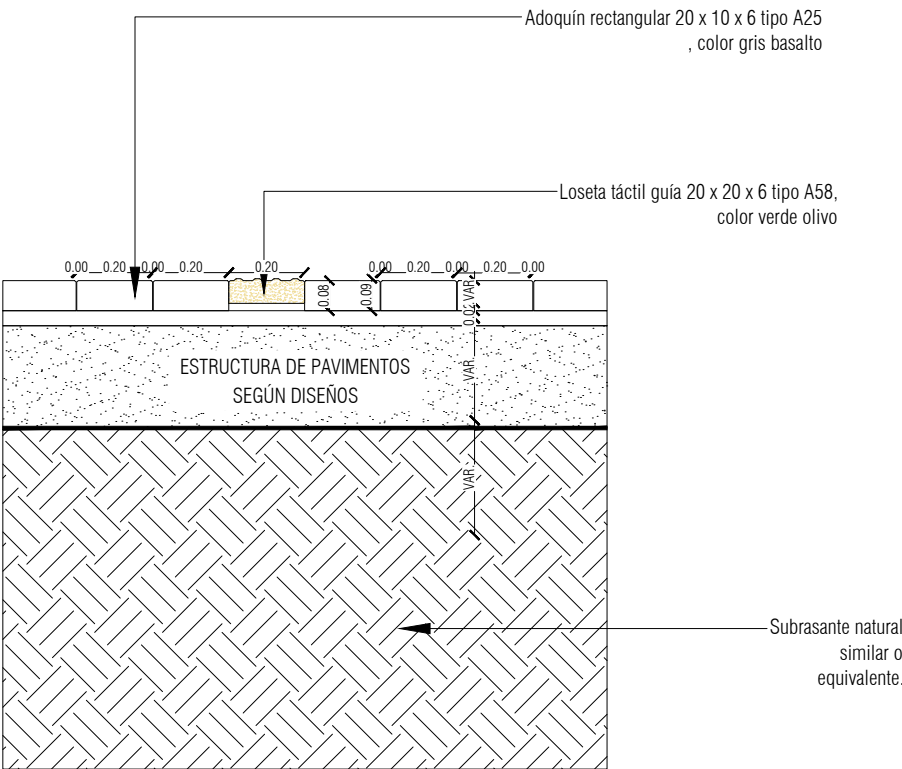
CORTE A-A LOSETA PREFABRICADA TÁCTIL GUÍA A-58 ESC: 1:20
