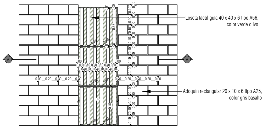
PLANTA LOSETA PREFABRICADA TÁCTIL GUÍA A-56 ESC: 1:20
