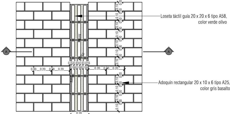
PLANTA LOSETA PREFABRICADA TÁCTIL GUÍA A-58 ESC: 1:20
