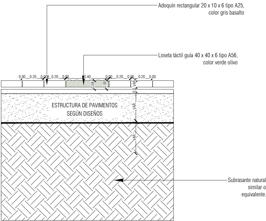
CORTE A-A LOSETA PREFABRICADA TÁCTIL GUÍA A-56 ESC: 1:20
