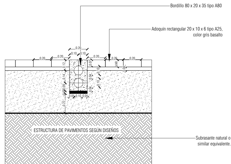
CORTE A-A DETALLE BORDILLO A-80 ESC: 1:20
