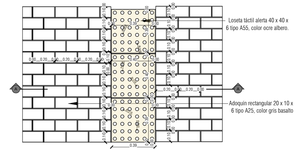
PLANTA DETALLE LOSETA TÁCTIL ALERTA A-55 ESC: 1:20
