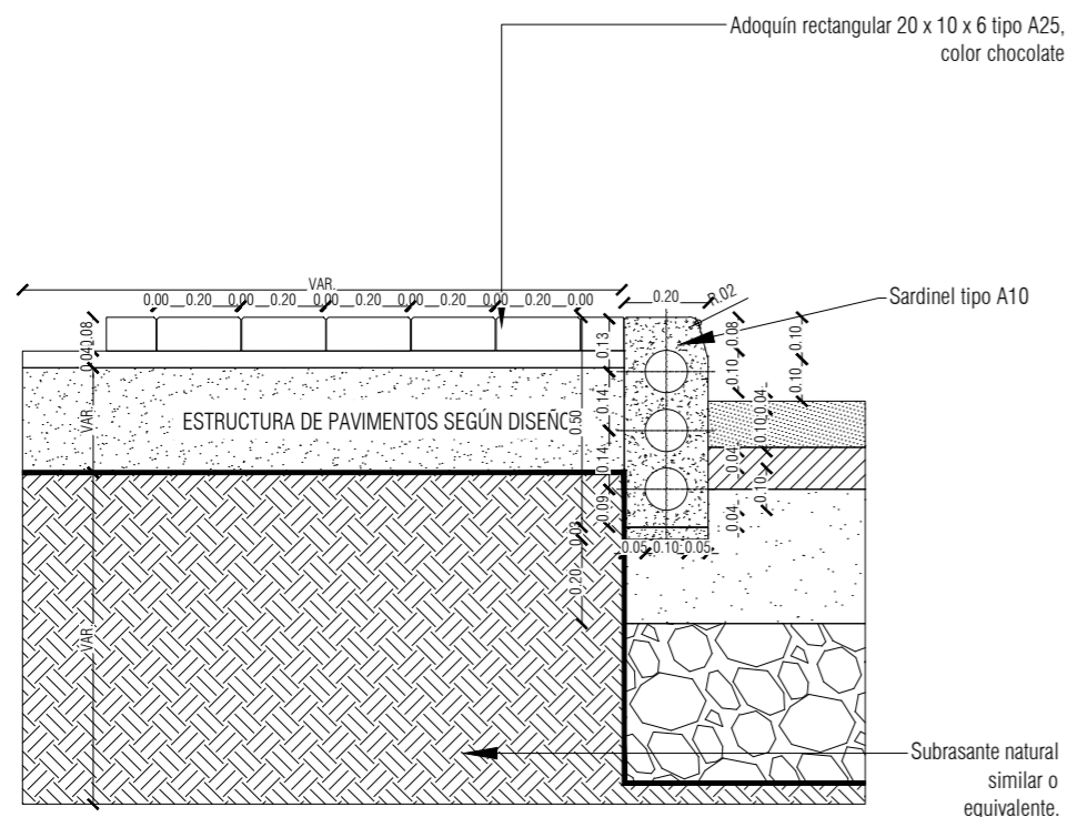
CORTE A-A DETALLE SARDINEL TIPO A-10 ESC: 1:20
