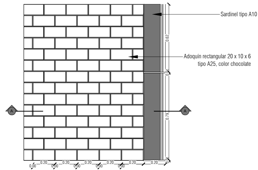
PLANTA DETALLE SARDINEL TIPO A-10 ESC: 1:20
