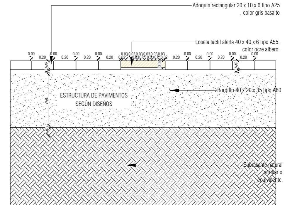
CORTE A-A DETALLE LOSETA TÁCTIL ALERTA TIPO A-55 ESC: 1:20
