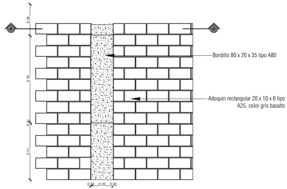
PLANTA DETALLE BORDILLO ESC: 1:20
