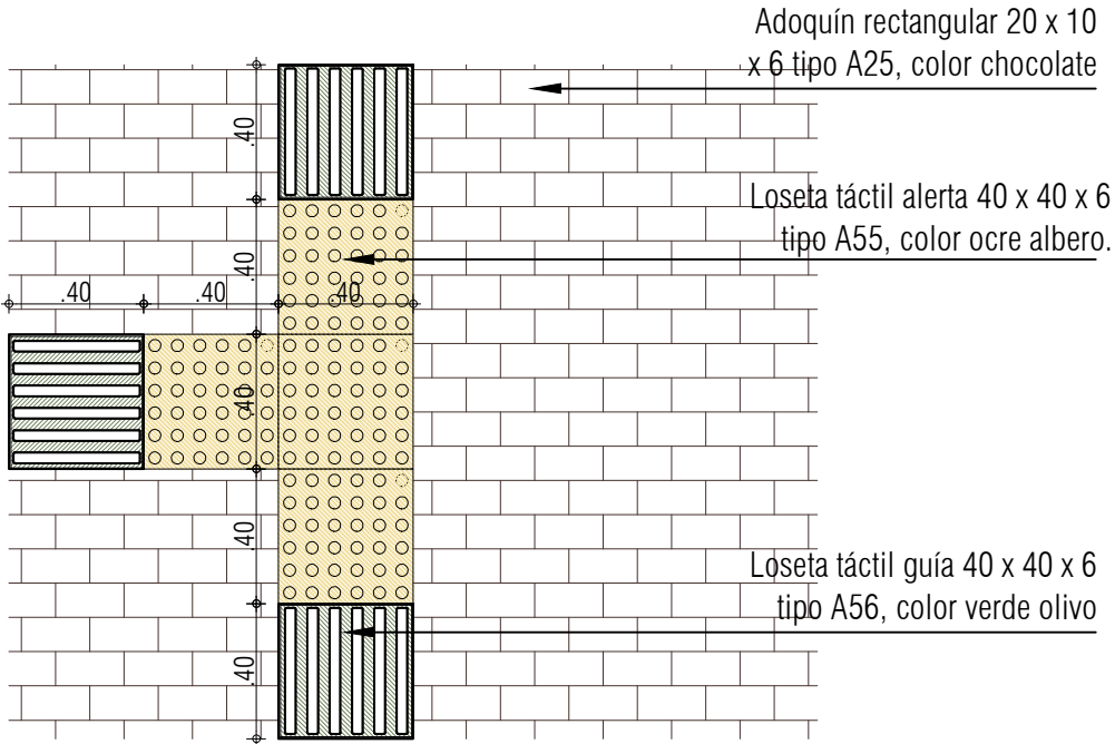
PLANTA PUNTO DE DECISIÓN EN T ESC: 1:25
