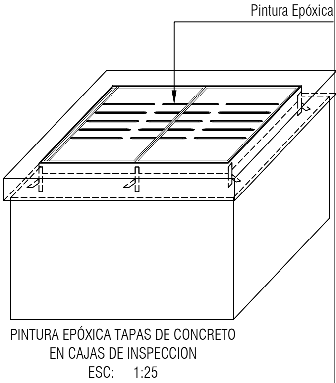
Pintura Epóxica PINTURA EPÓXICA TAPAS DE C EN CAJAS DE INSPECC ESC: 1:25
