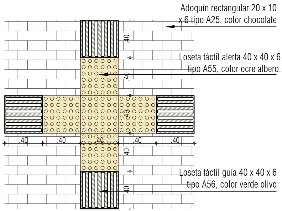
PLANTA PUNTO DE DECISIÓN EN CRUZ ESC: 1:25
