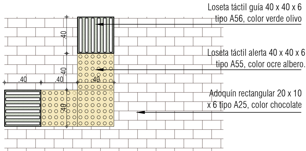
PLANTA PUNTO DE DECISIÓN EN L ESC: 1:25
