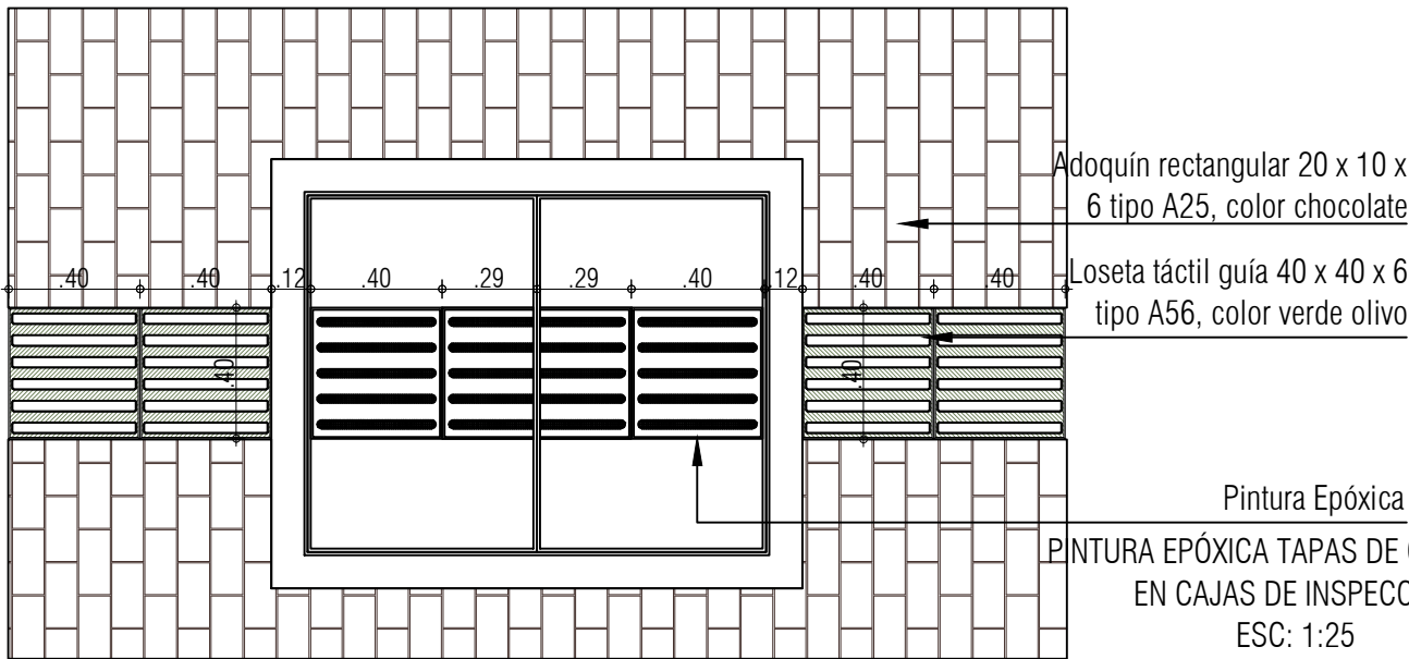
PLANTA PUNTO DE DECISIÓN EN T ESC: 1:25
