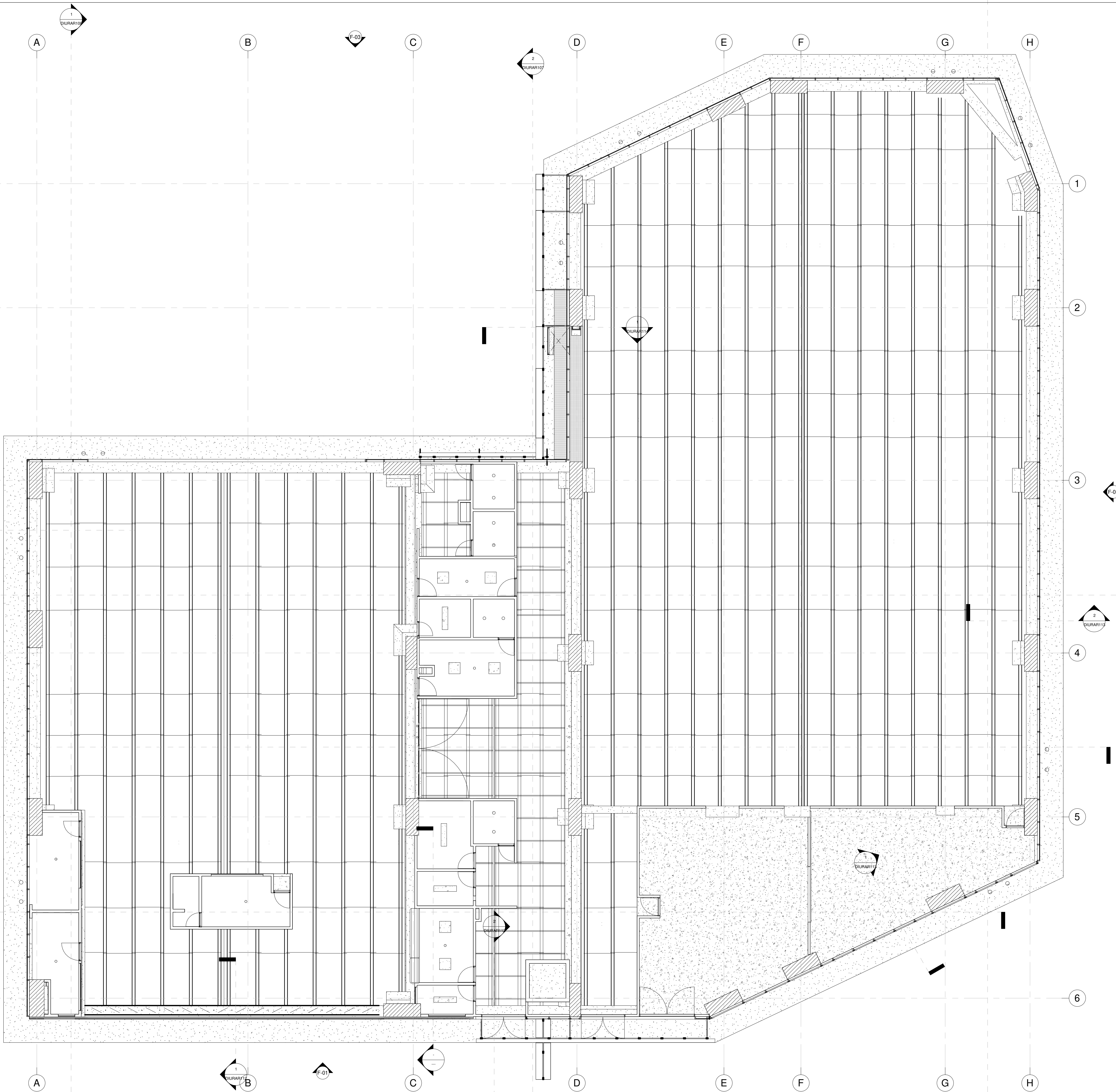
1 Planta 05_PLANTA CIELO RASO_ABORDAJE 1 : 100
