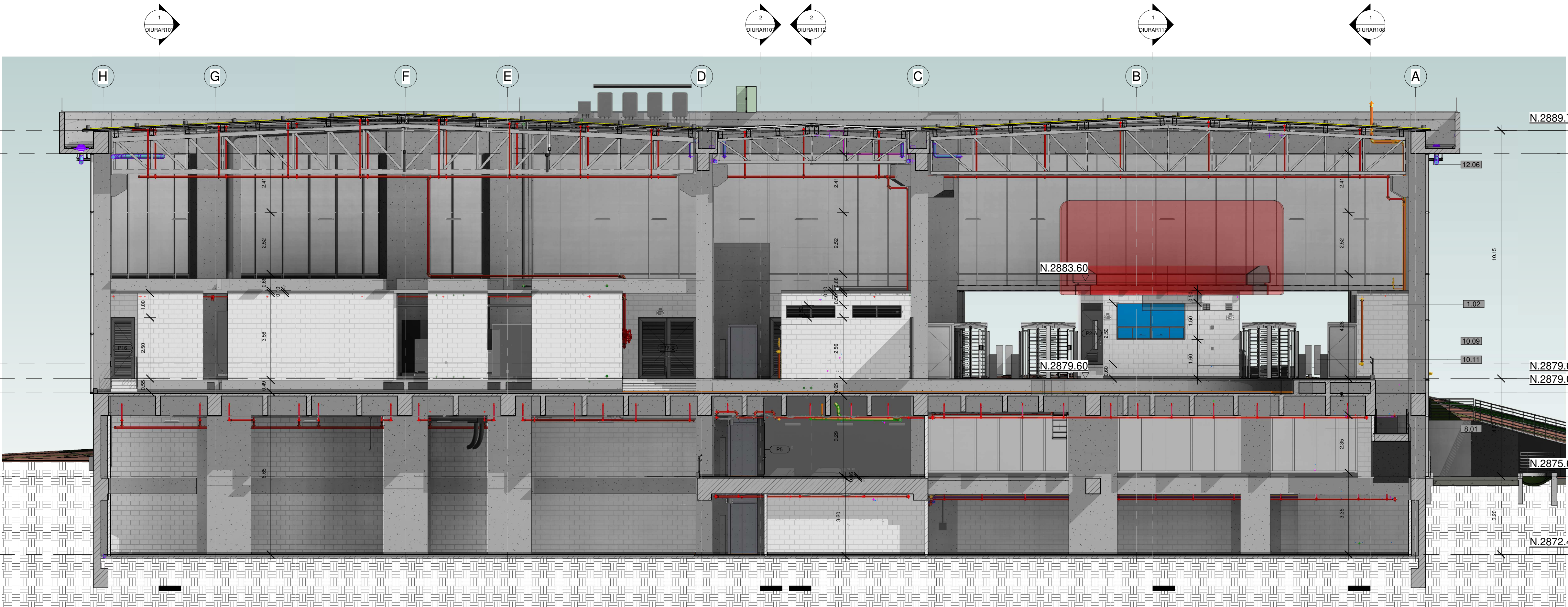
2 CORTE-06 1 : 100
