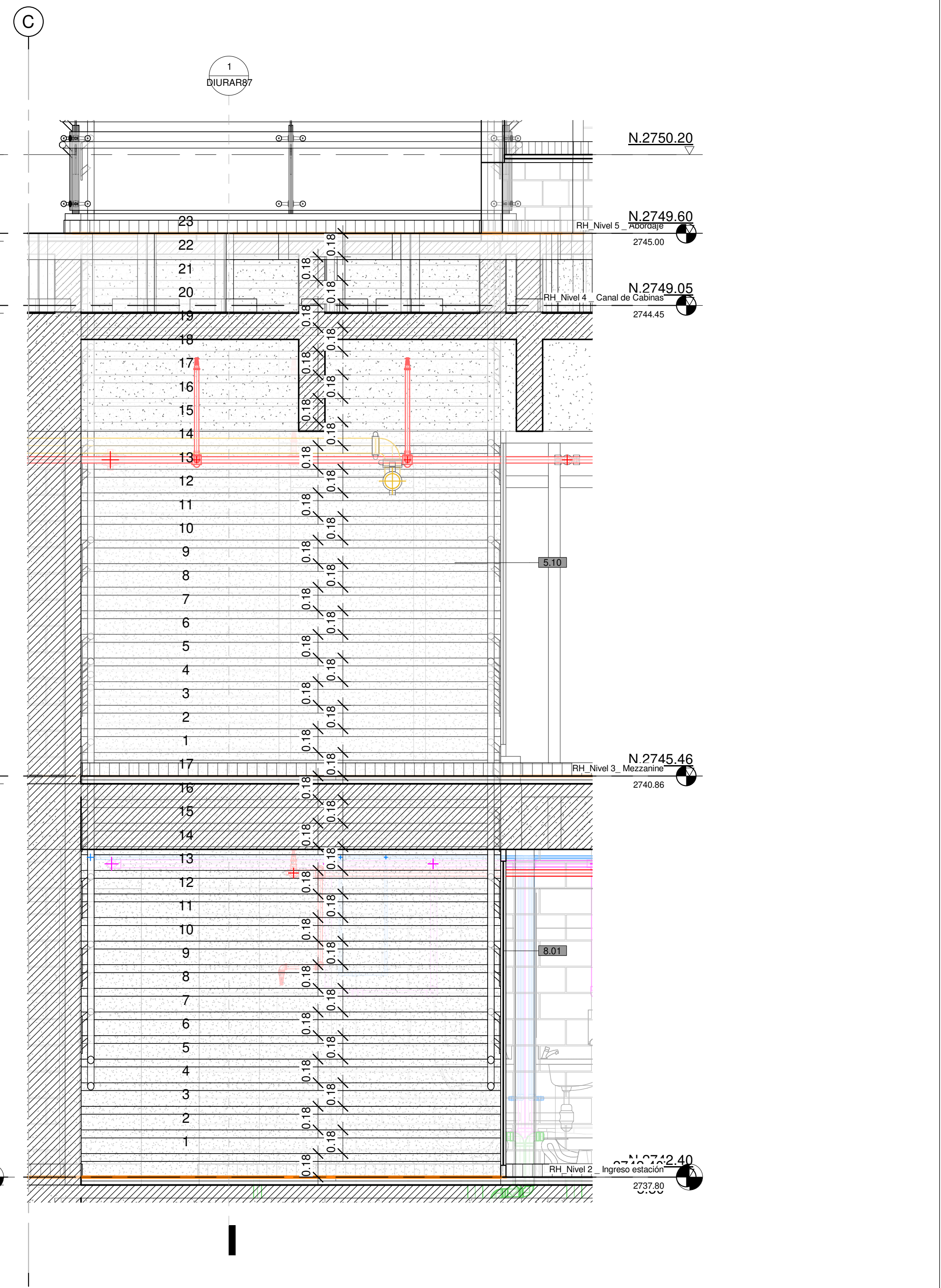
2 ESCALERA TIPO 02_ES2_CORTE 02 1 : 25
