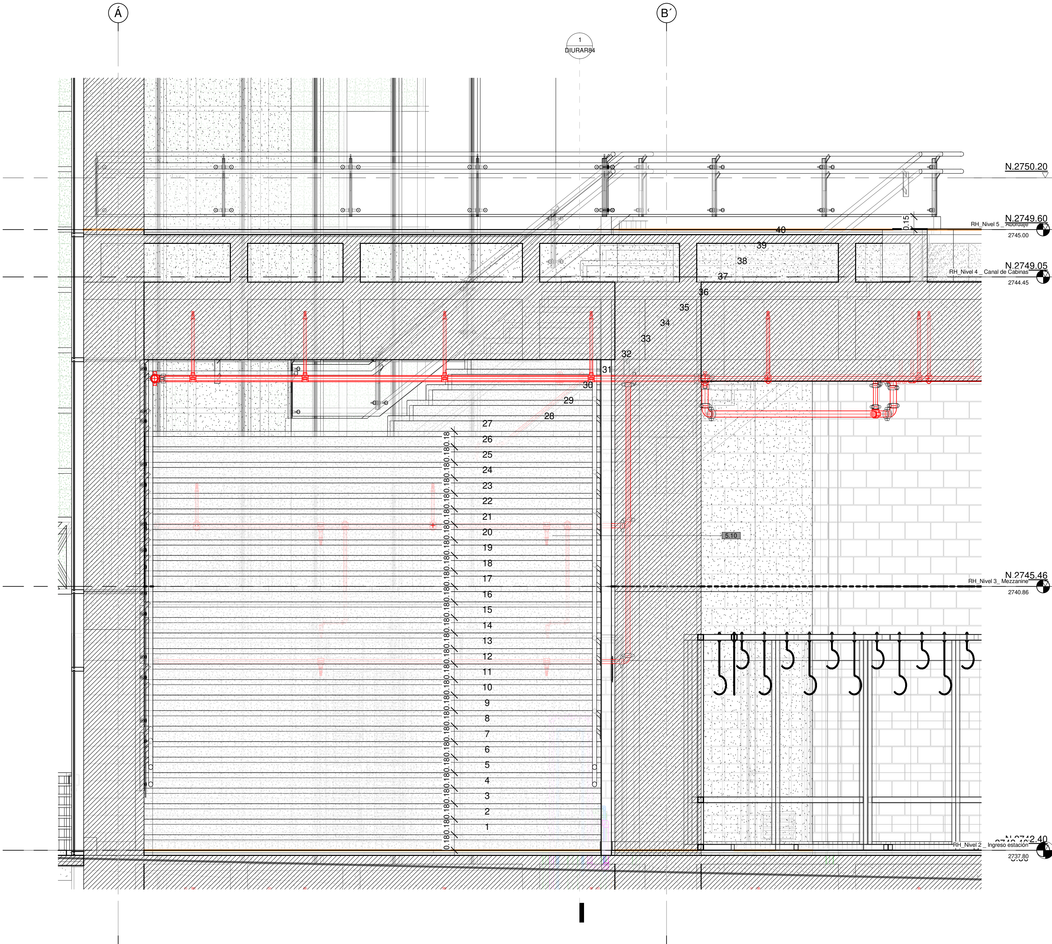
1 ESCALERA TIPO 01_ES2_CORTE 02 1 : 25
