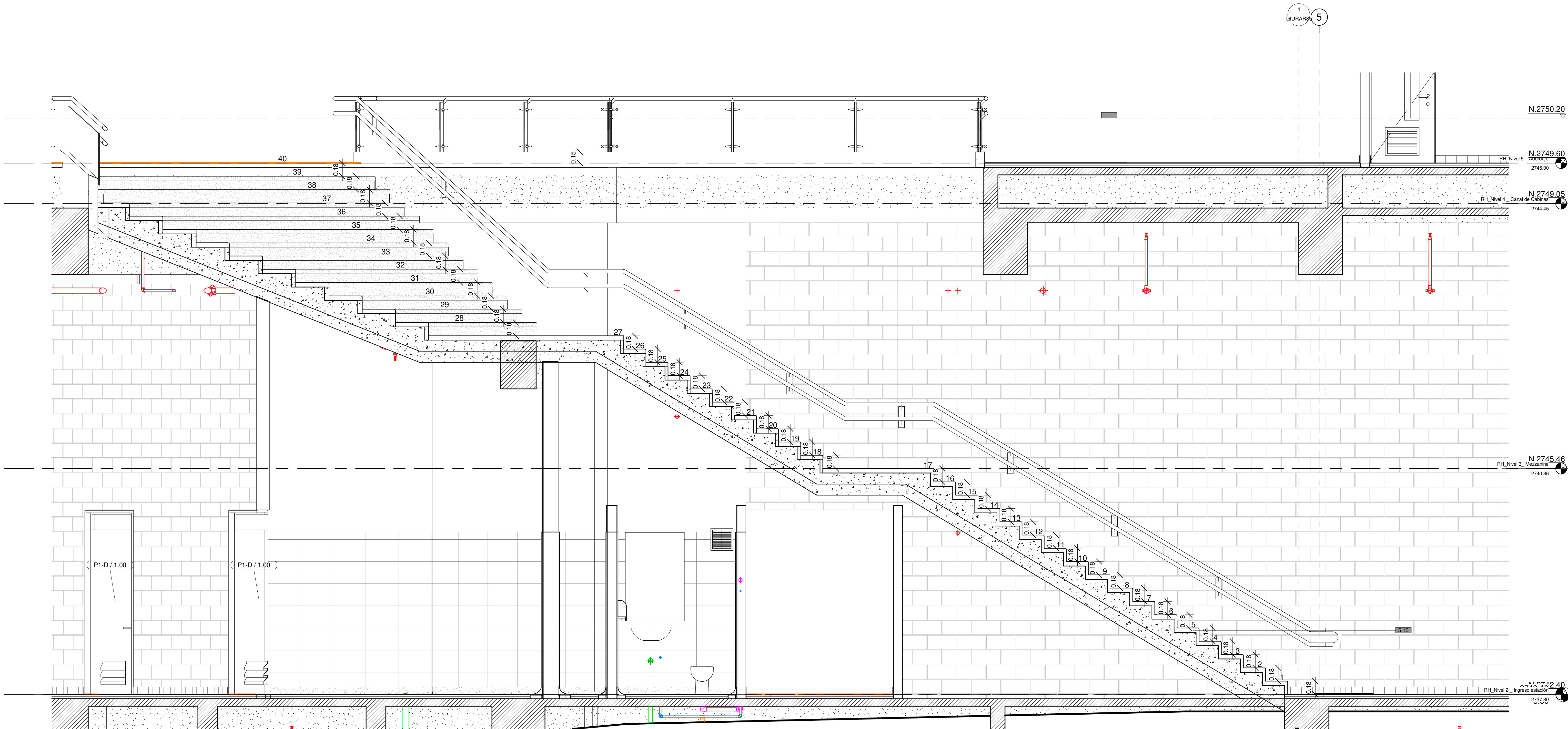
1 ESCALERA TIPO 01_ES2_CORTE 01 1 : 25
