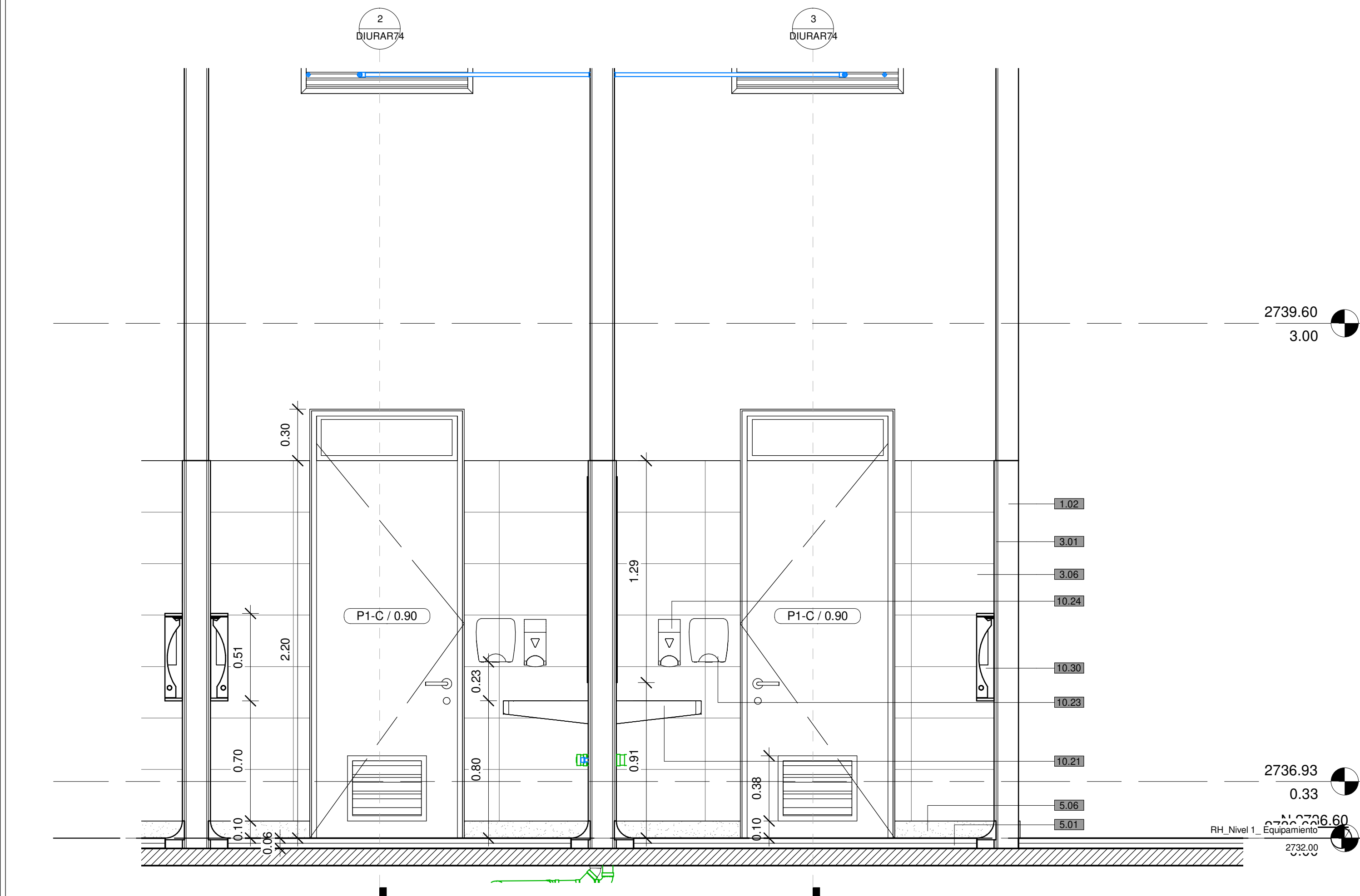
4 BAÑO TIPO 02_CORTE 03 1 : 20
