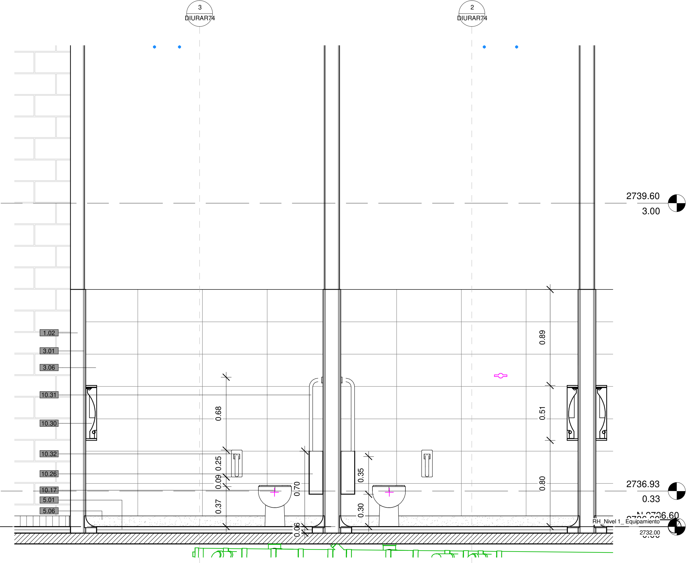
5 BAÑO TIPO 02_CORTE 04 1 : 20
