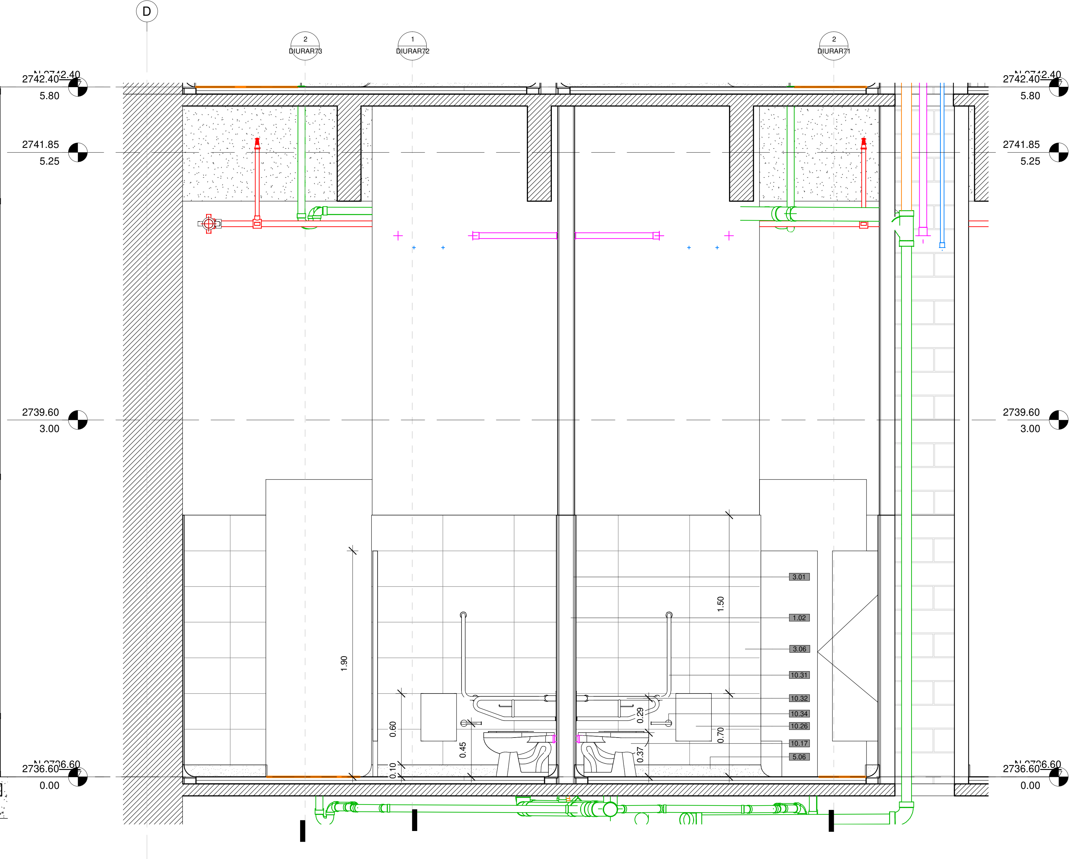
2 BAÑO TIPO 01_CORTE 03 1 : 20
