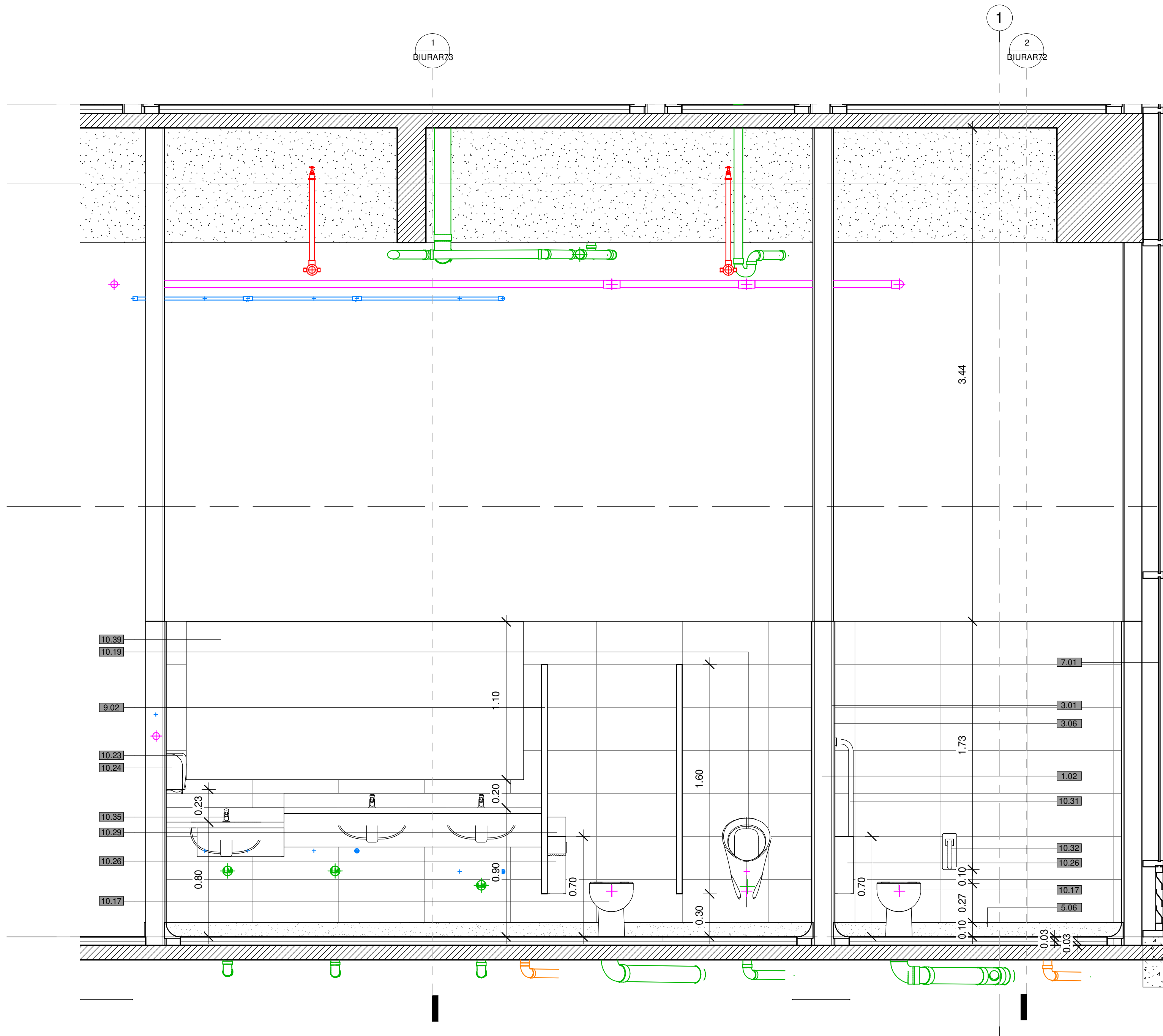
1 BAÑO TIPO 01_CORTE 02 1 : 20
