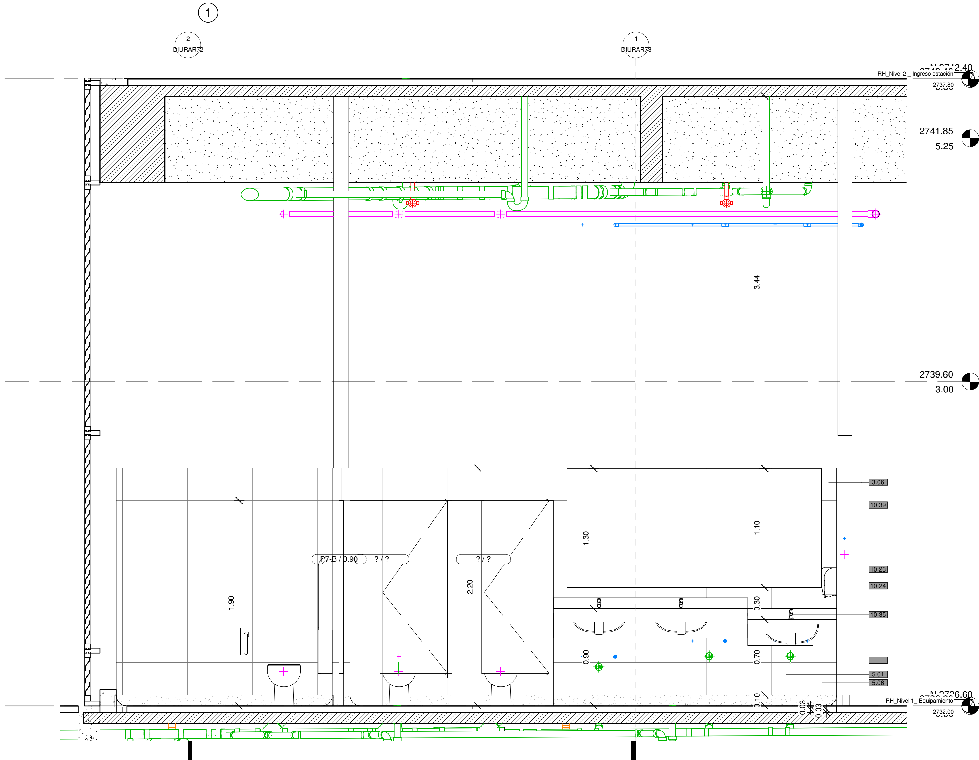
BAÑO TIPO 01_CORTE 01 1 : 20
