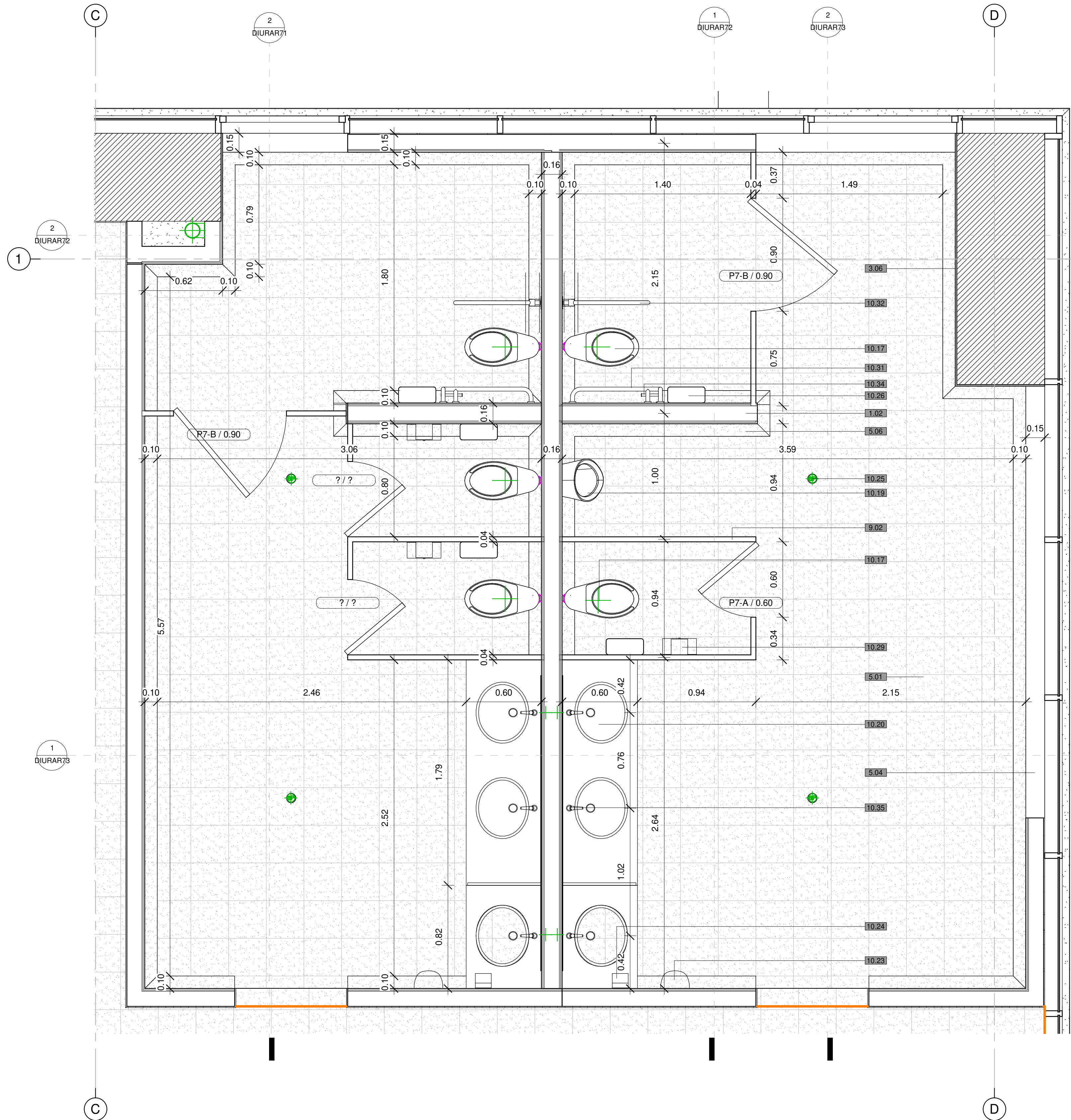
BAÑO TIPO 01 1 : 20
