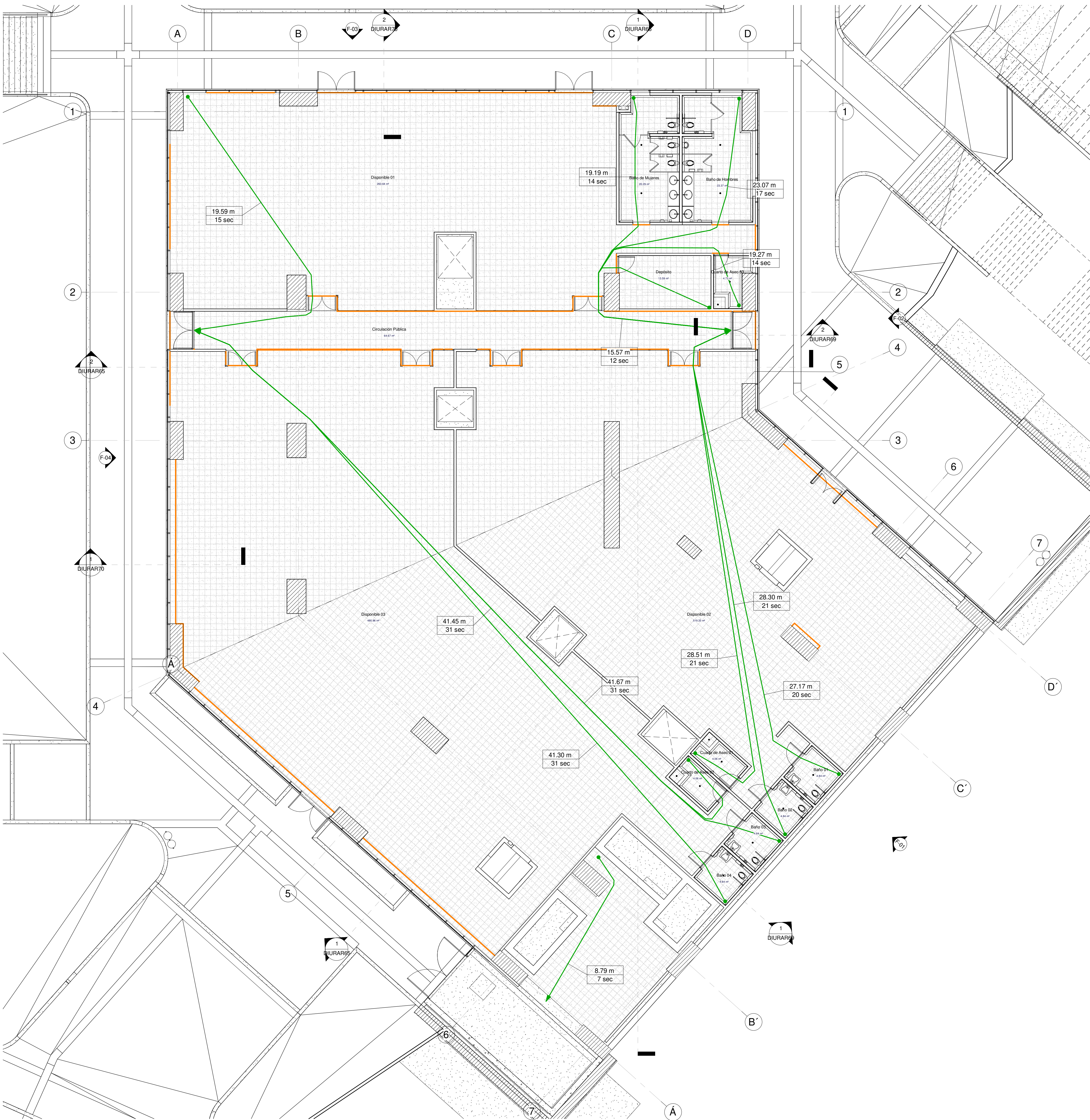
1 Planta 15_ RUTA DE EVACUACIÓN EQUIPAMIENTO 1 : 100
