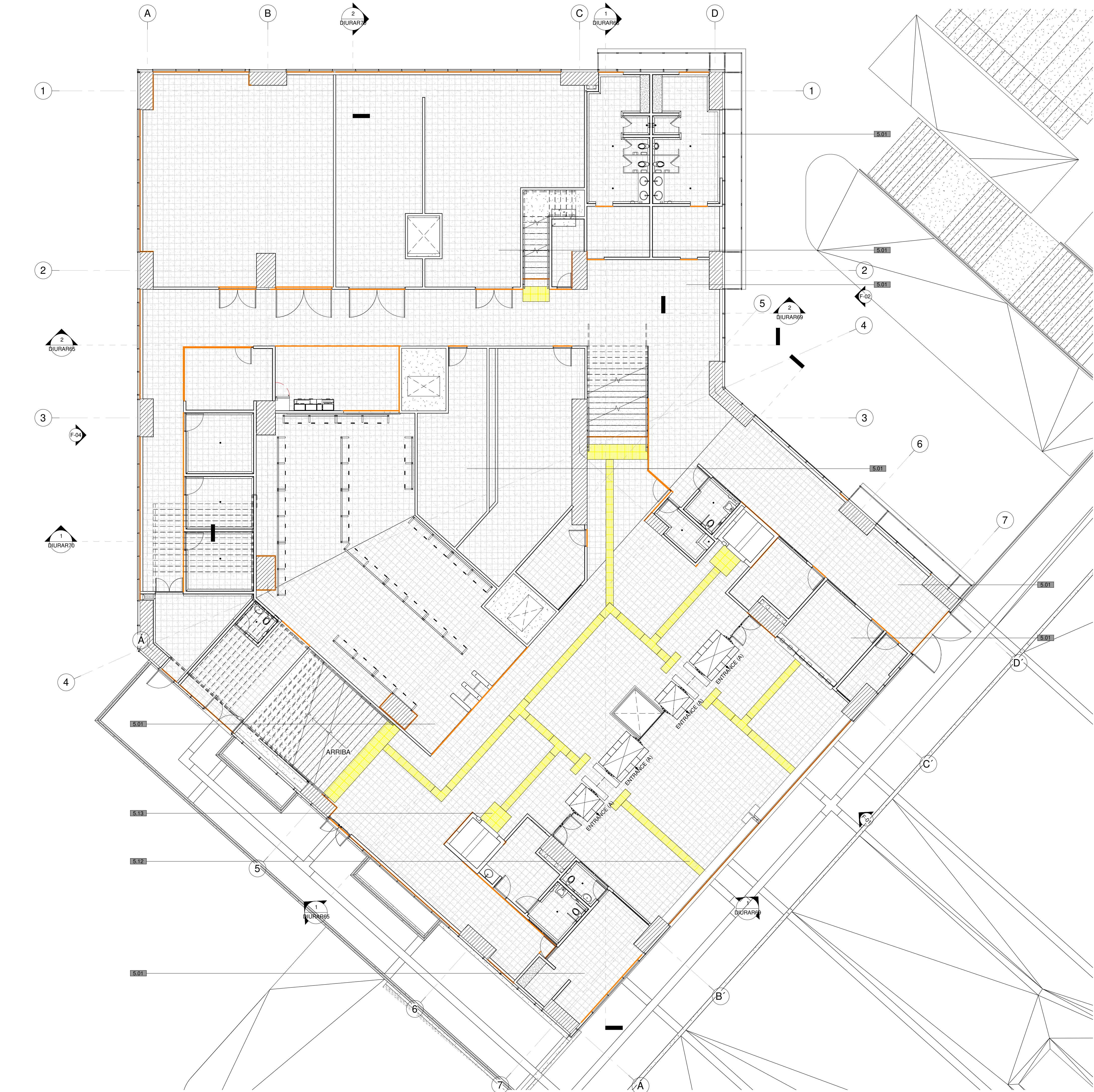
1 Planta 12_ DESPIECES DE PISOS_INGRESO ESTACIÓN 1 : 100
