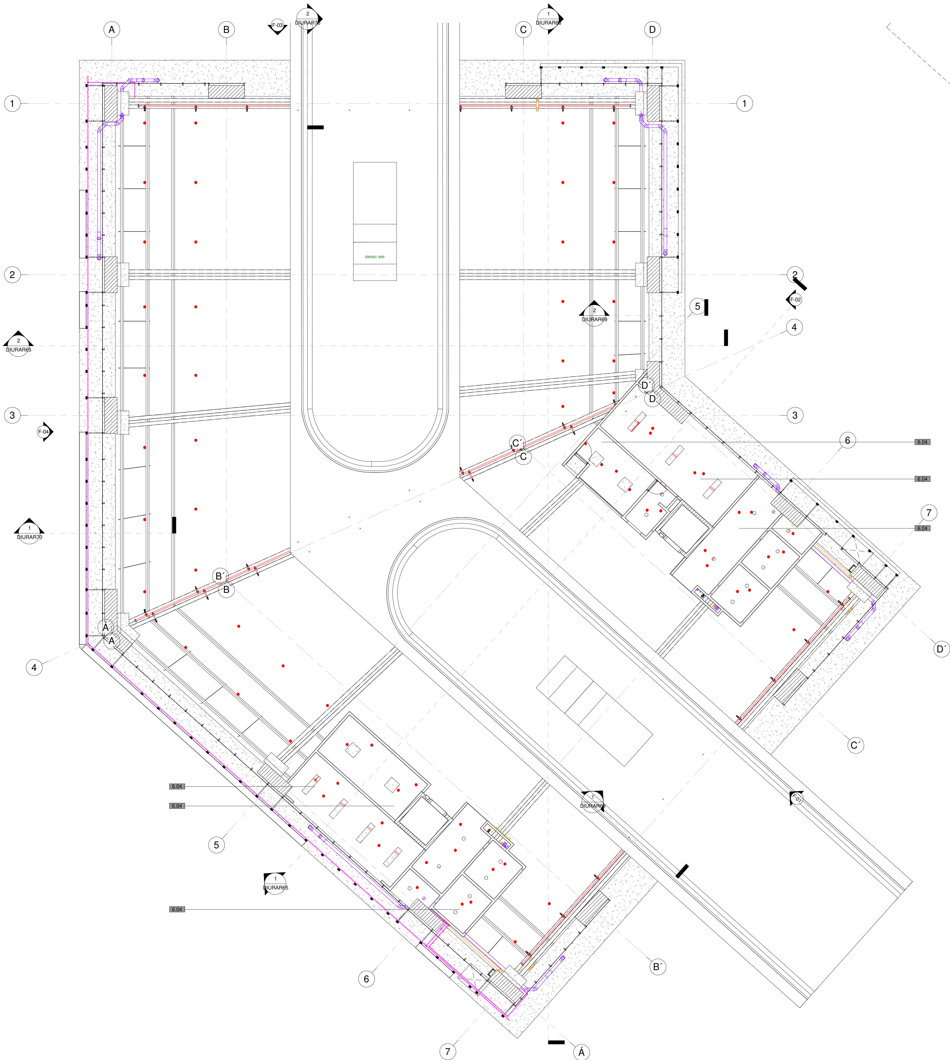
1 Planta 06 _ CIELO RASO_ Abordaje 1 : 100
