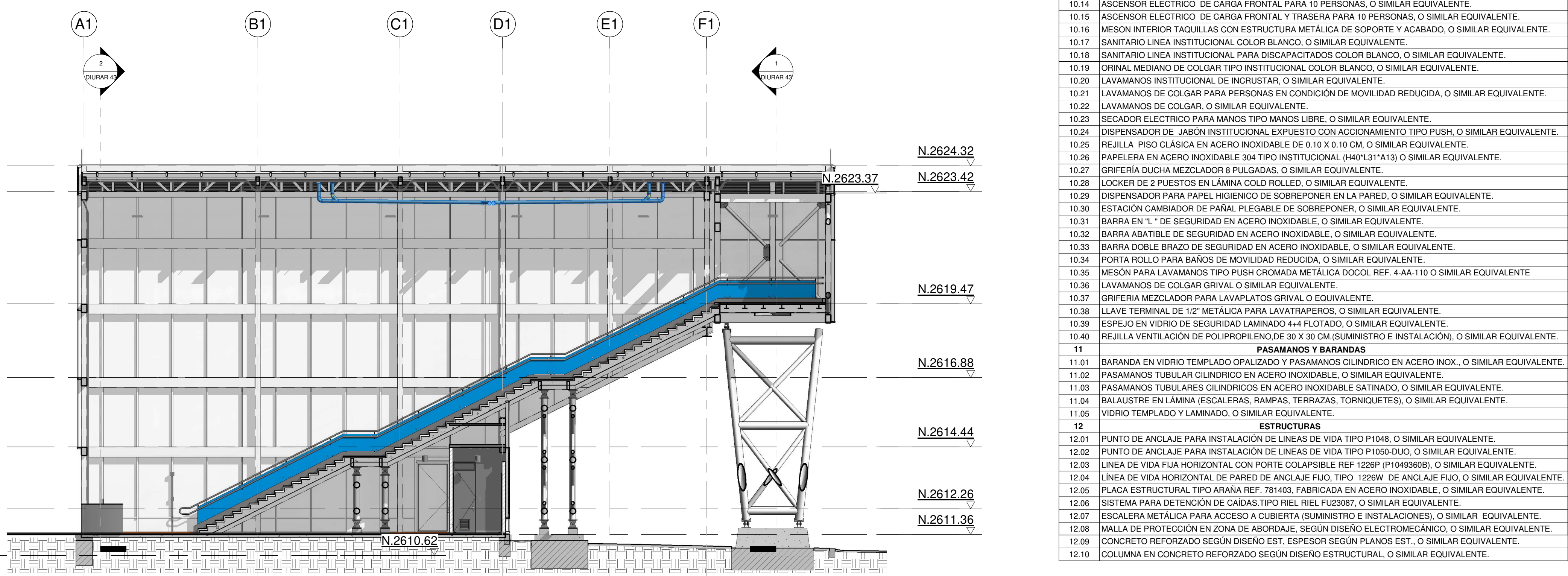
3 CORTE PUENTE-03
