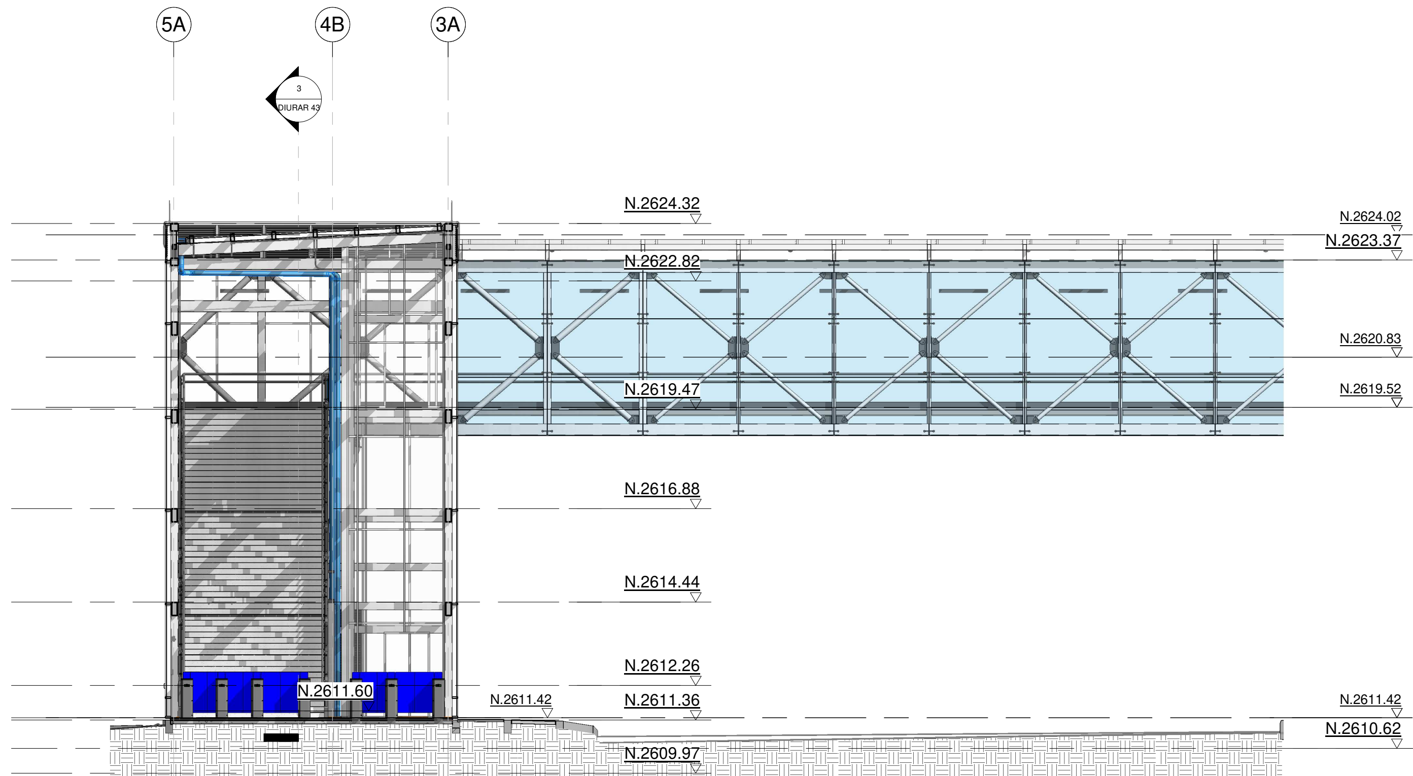
1 CORTE PUENTE-01
