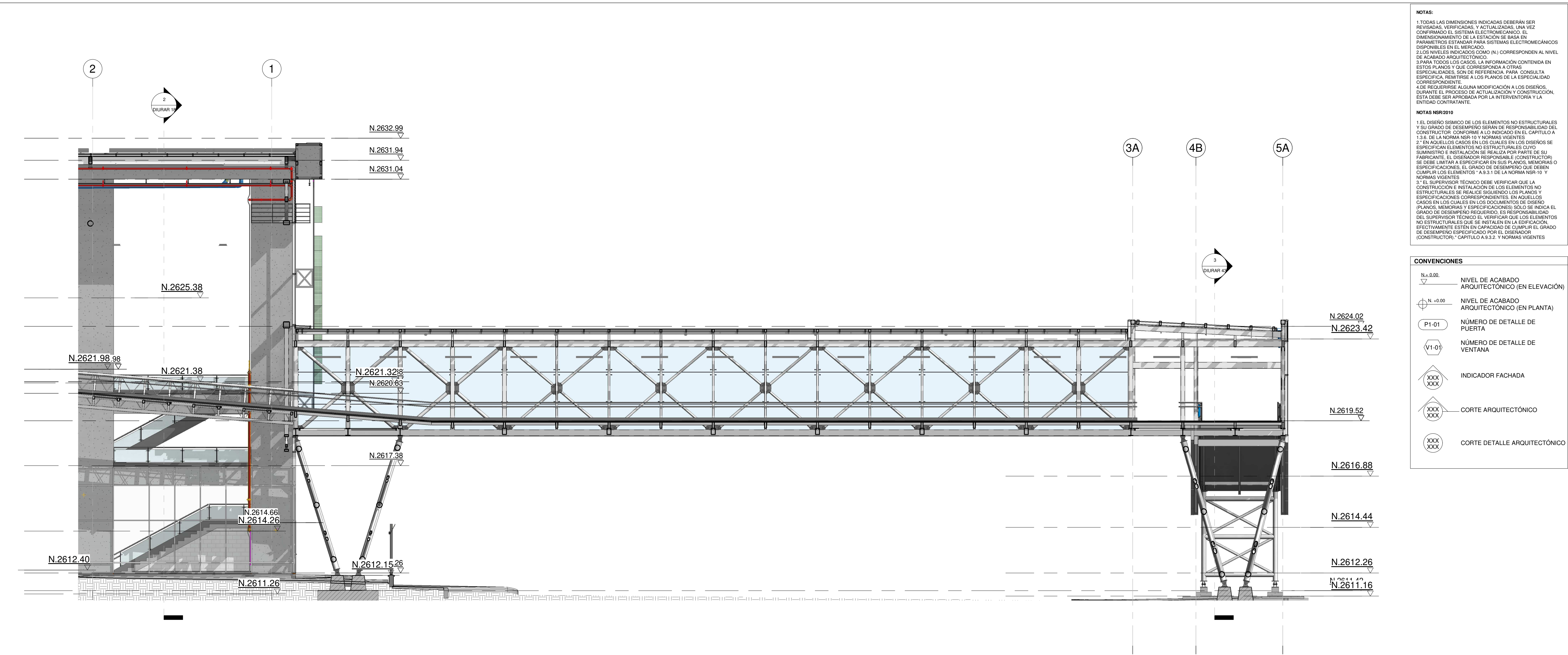
1 CORTE PUENTE-01
