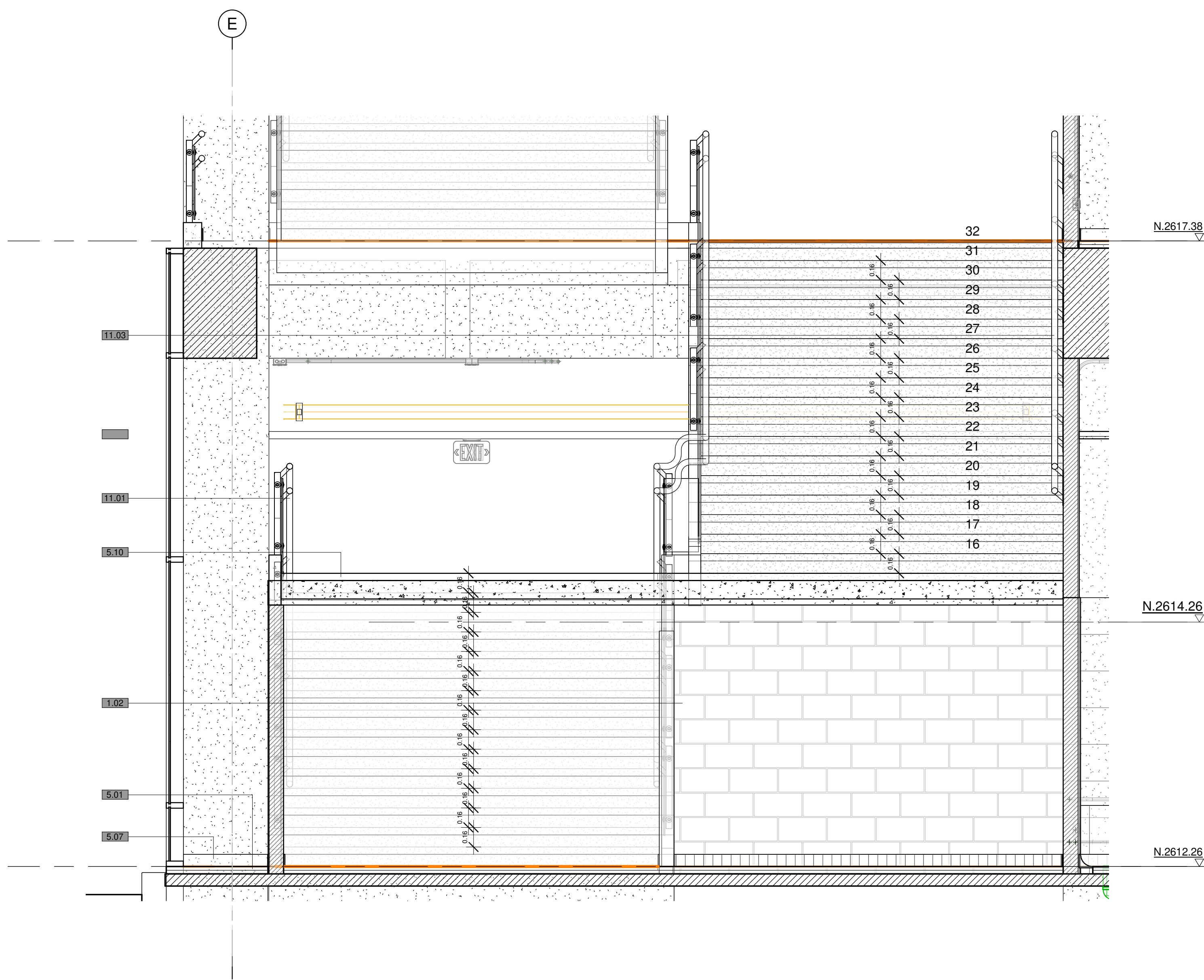
2 ESCALERA TIPO 01_ES1_CORTE 03 1 : 25
