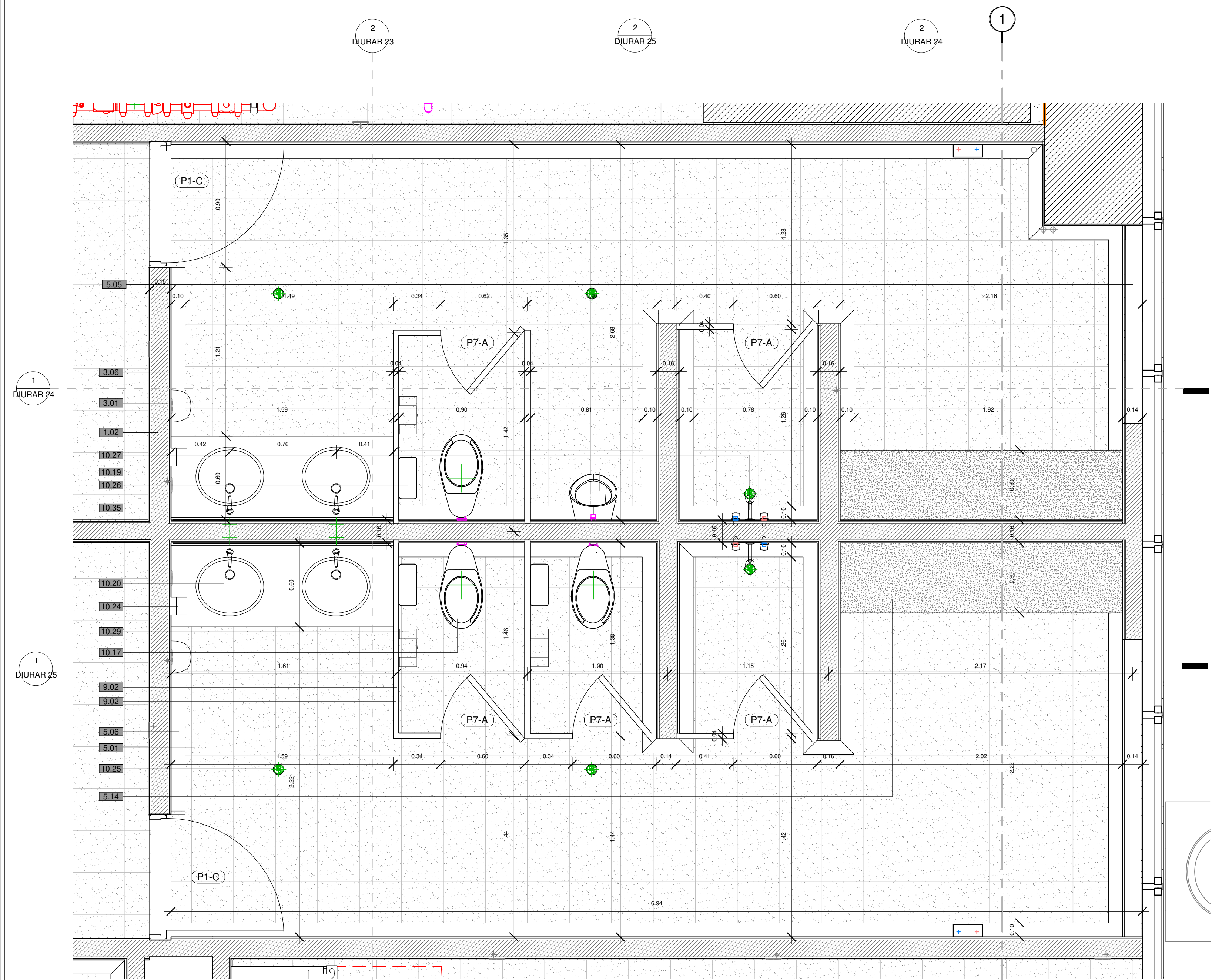
1 BAÑO TIPO 01 1 : 20
