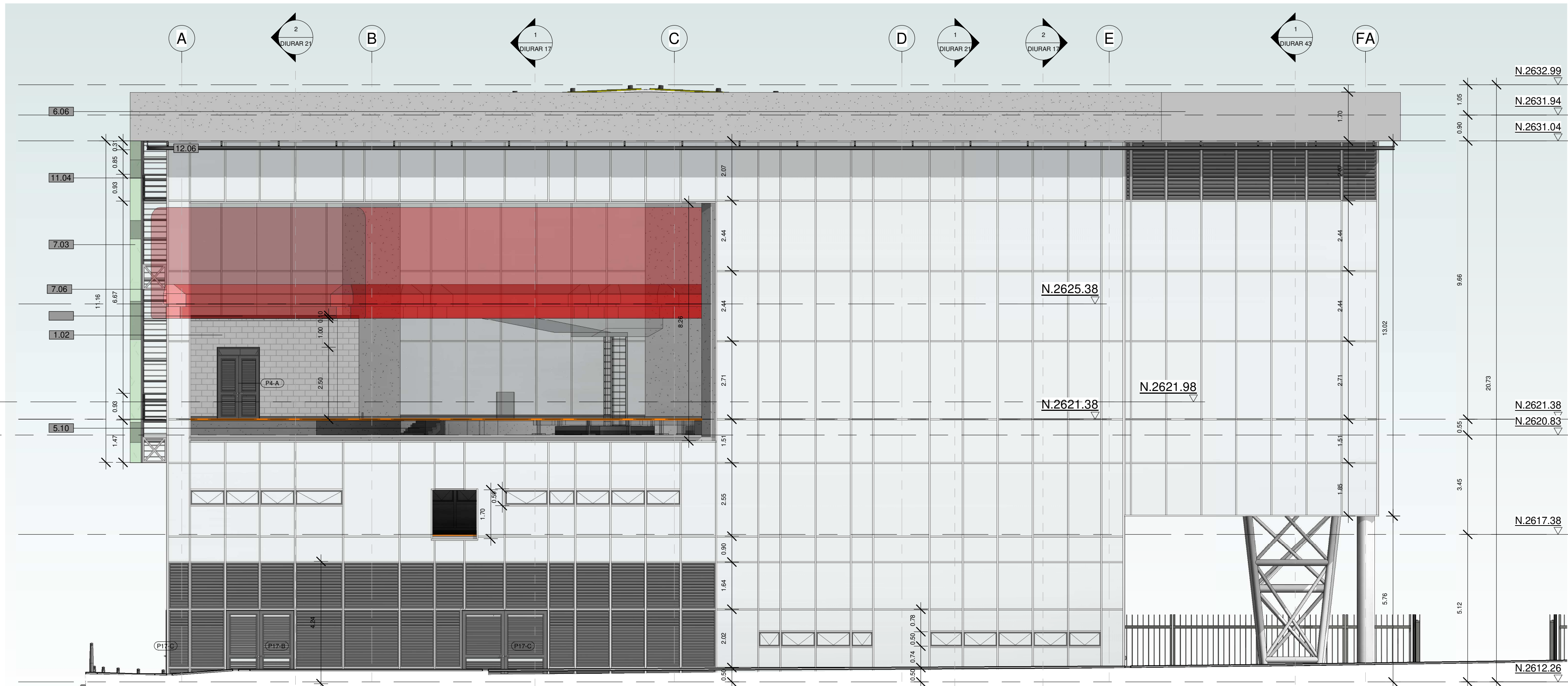
1 F-01 1 : 100
