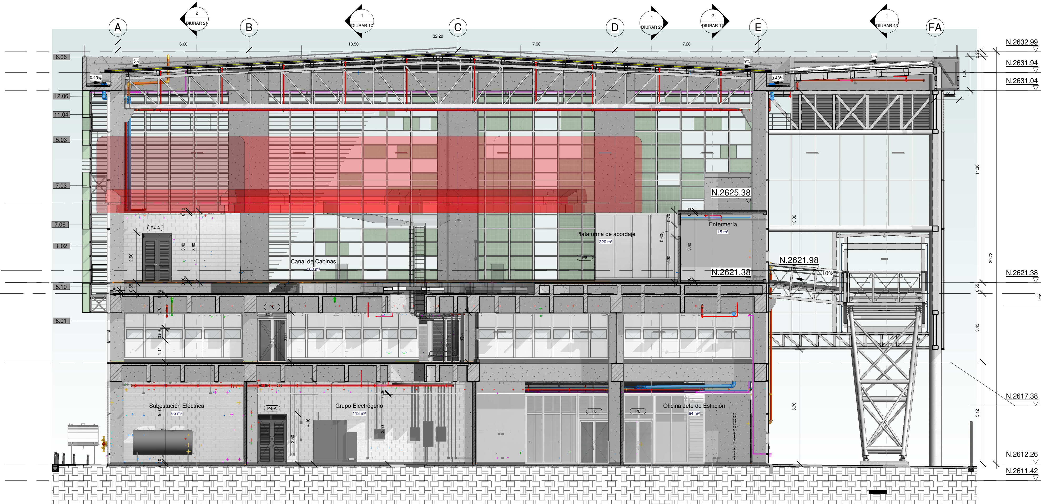
1 CORTE-03 1 : 100
