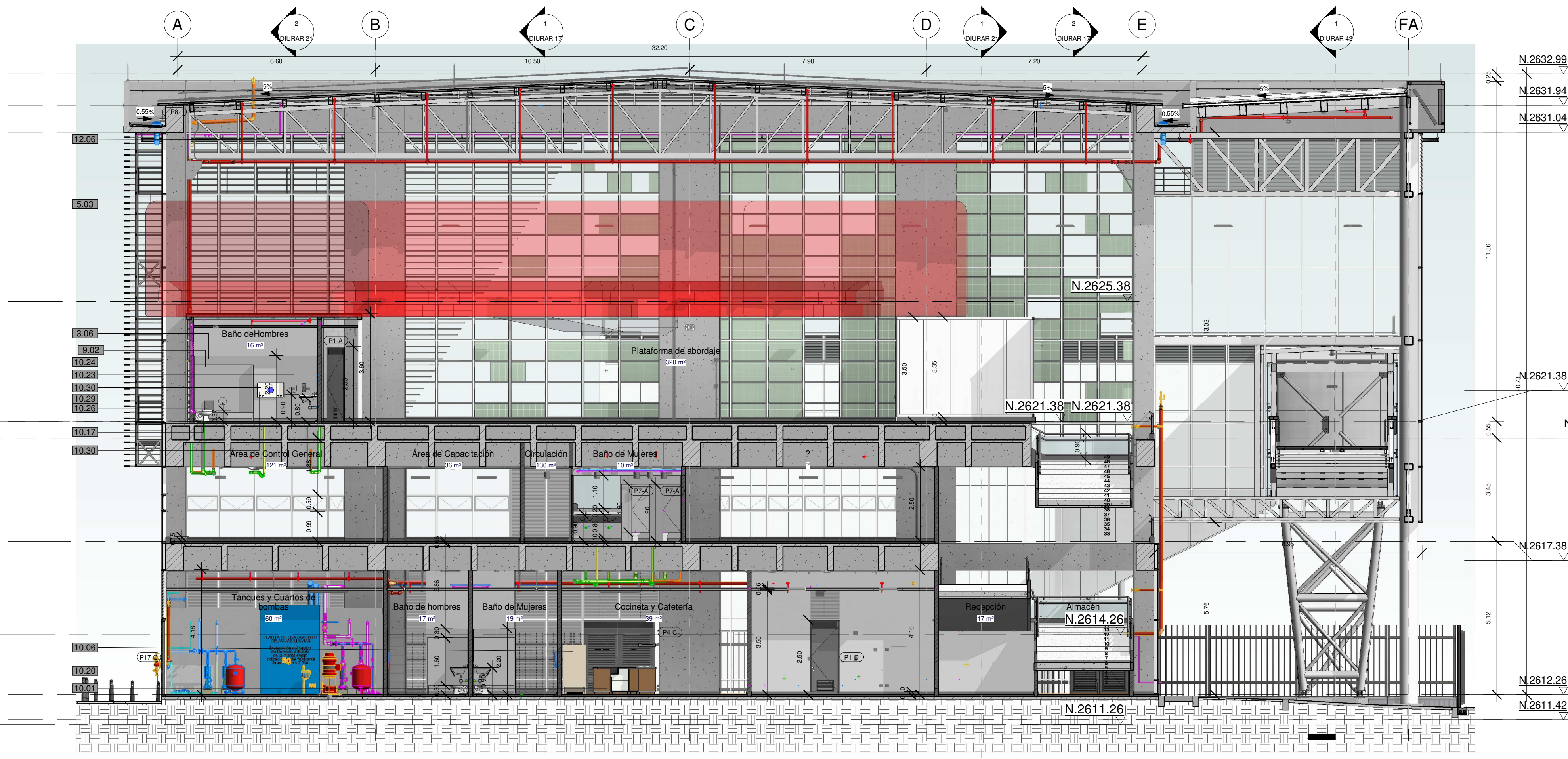
2 CORTE-04 1 : 100
