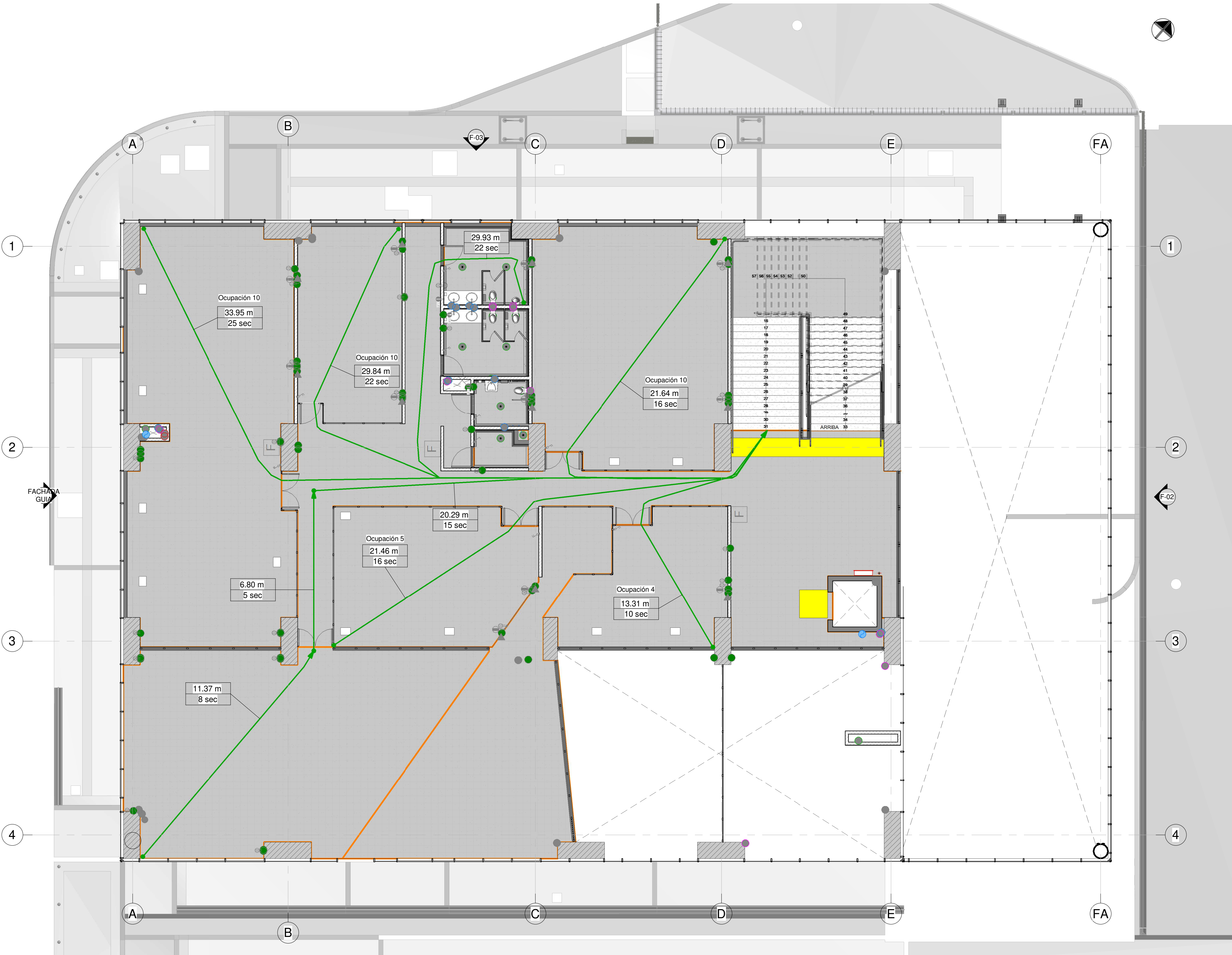
1 Planta 14_RUTA DE EVACUACIÓN_MEZZANINE 1 : 100
