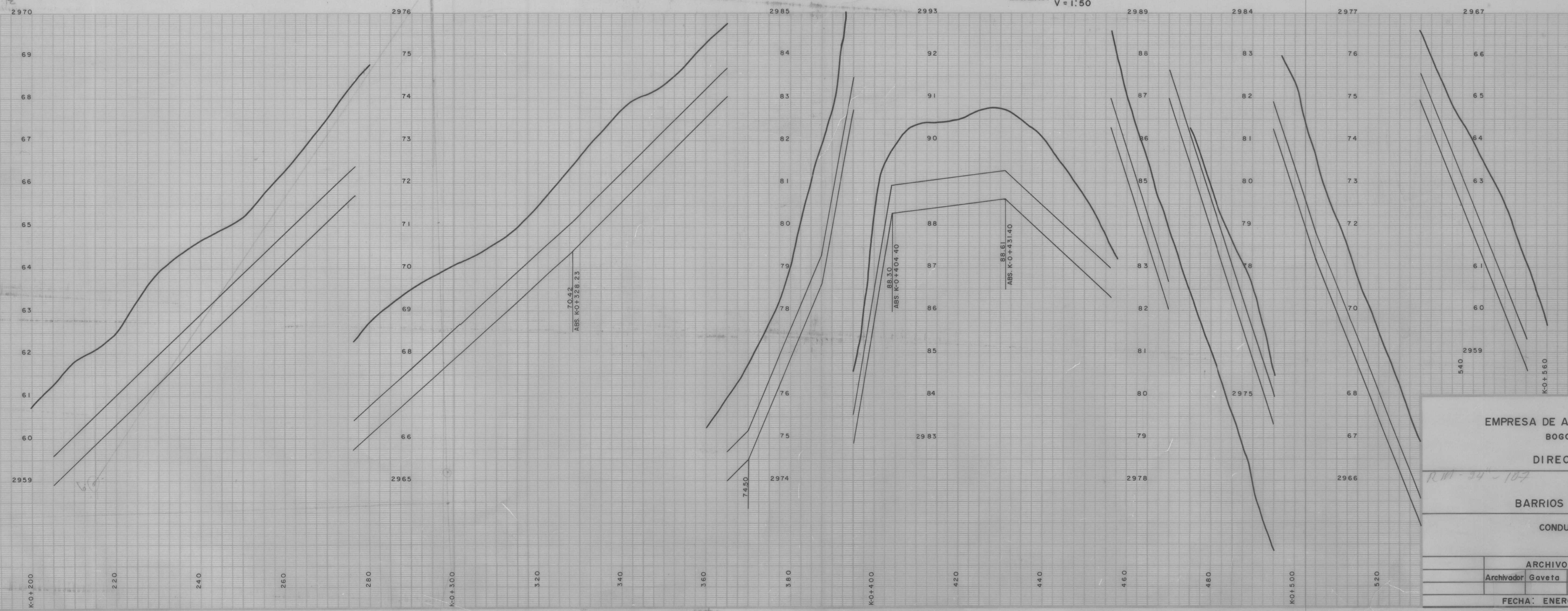
PERFIL ESCALAS: H=1:500 V=1:50
