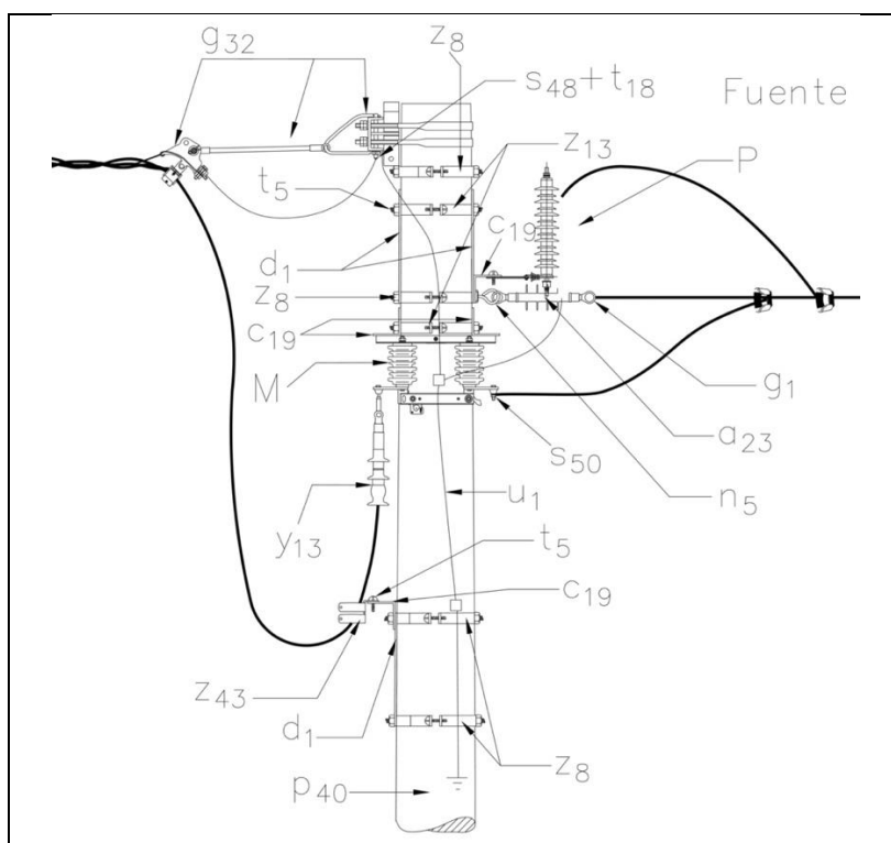
Figura 7 - Estructura LA655-Transición a desnudo
