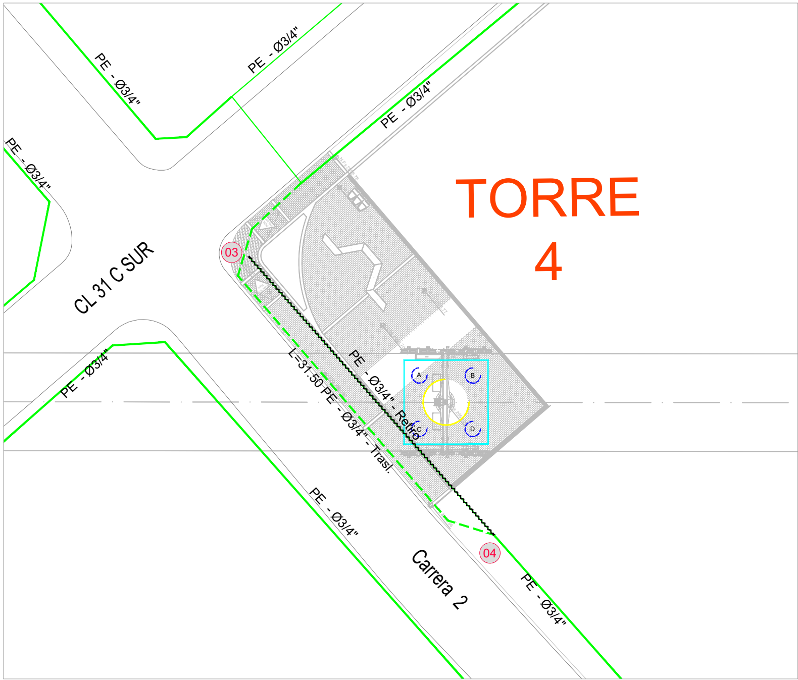
DETALLE PILONA 4 ESCALA: 1:250
