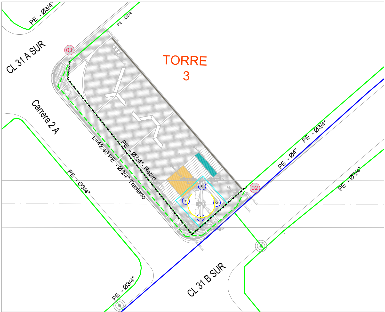
DETALLE PILONA 3 ESCALA: 1:250
