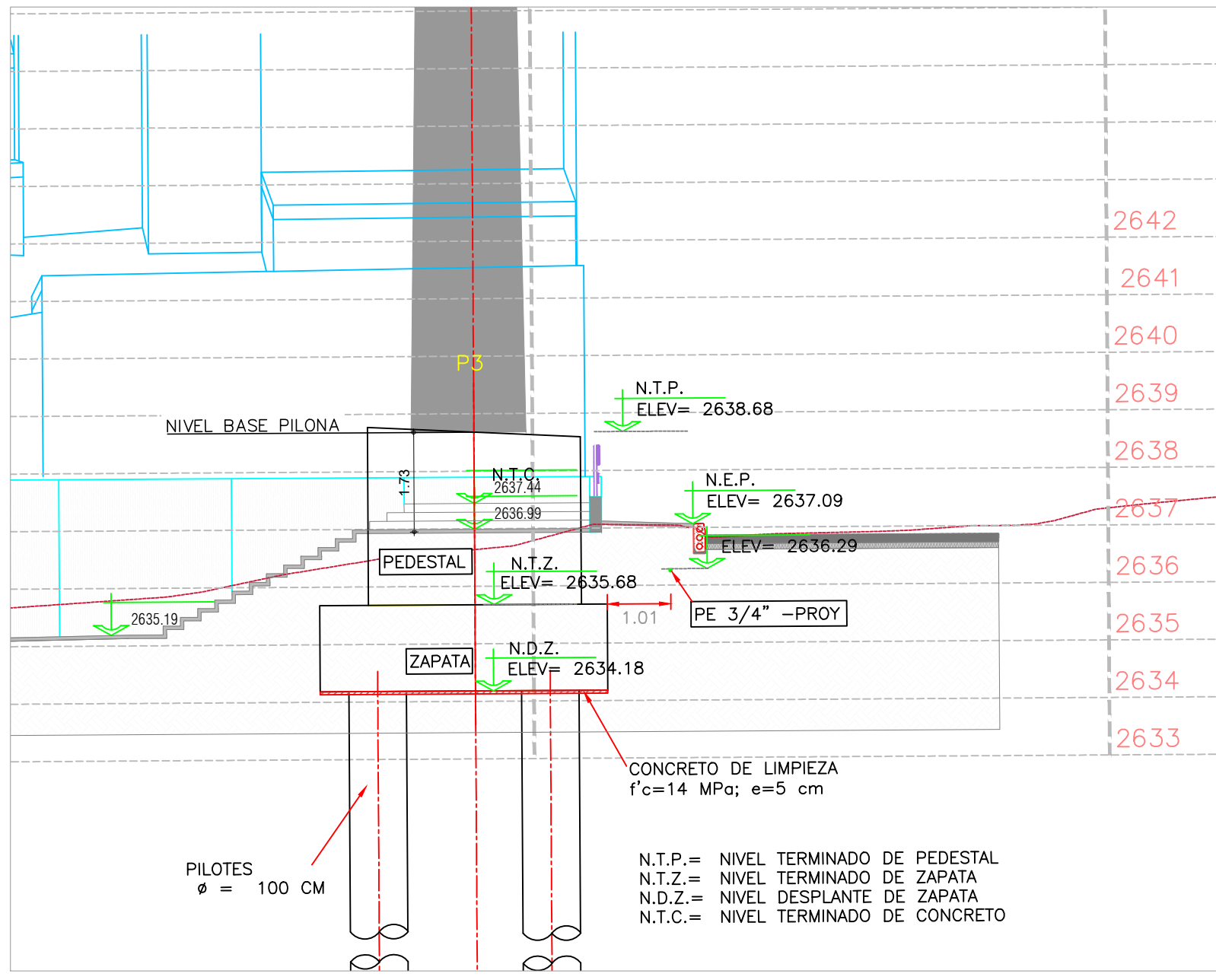
CORTE A-A (CIMENTACIÓN PILONA 3) ESCALA: 1:100
